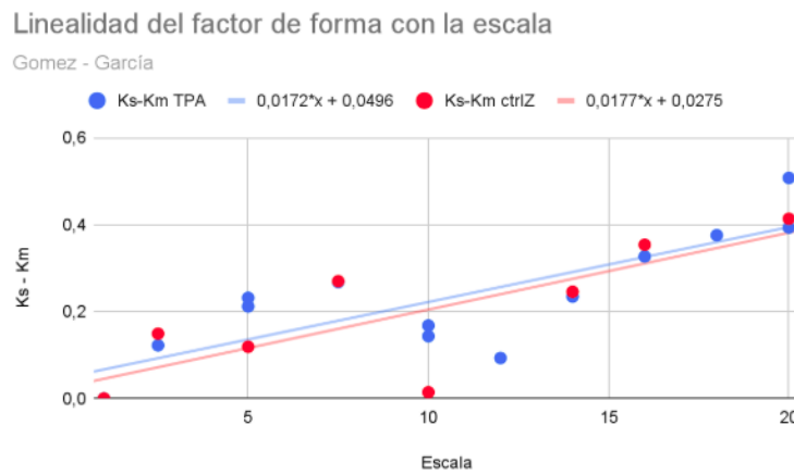
Figura 4.1.24: Linealidad del factor de forma con la escala para el P1 , siguiendo el método de Garcia-Gómez [2000].
