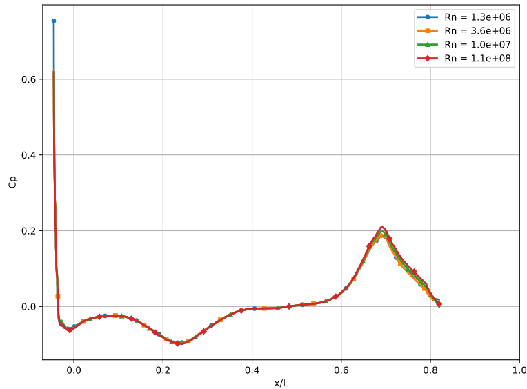
Figura 4.1.35: Distribución de C_P(x/L) sobre el plano z/T = 0,75 .
