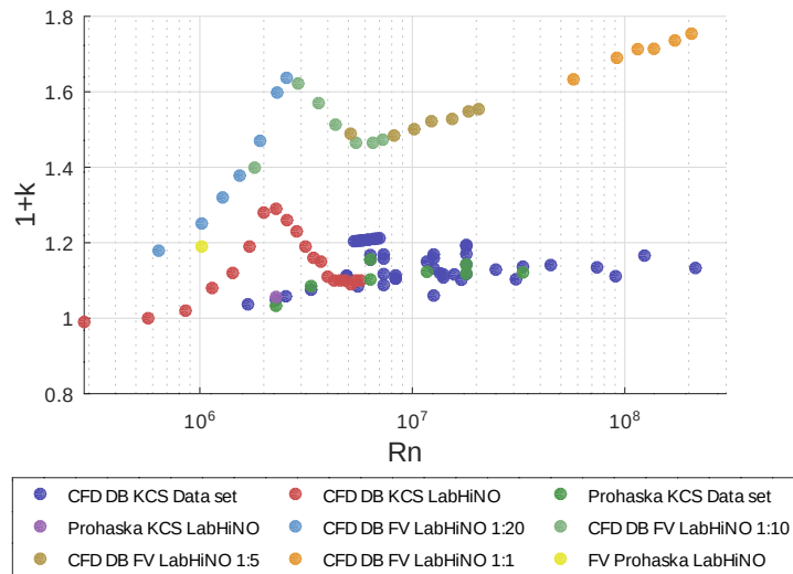
Figura 4.1.22: (1+k) frente a R_n para el KCS y el P1, en escala logarítmica. Para el KCS se muestran los resultados propios obtenidos en el LabHiNO (CFD DB y Prohaska EFD, escala 1:79) junto con el conjunto de datos recopilado por Terziev et al. [2020] (CFD DB y Prohaska, otras escalas y laboratorios). Para el P1 se muestran únicamente resultados propios: CFD DB en las escalas 1:20, 1:10, 1:5 y 1:1, y el valor experimental obtenido por Prohaska en el LabHiNO (escala 1:20).
