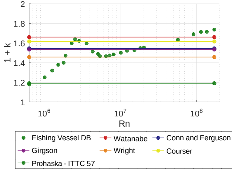
Figura 4.6.1: Valores de (1 + k) para el P1 en función de R_n , obtenidos por CFD DB, EFD y correlaciones empíricas de la literatura [Molland et al., 2017, Conn and Ferguson, 1968, Grigson, 2000, Wright, 1984, Couser et al., 1997].
