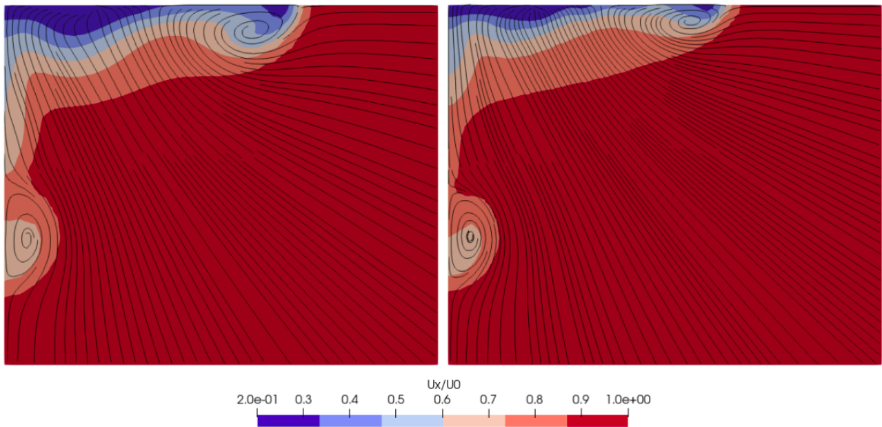
Figura 4.1.27: Contornos de velocidad longitudinal U_x/U_0 en un plano ubicado en x/L = 0,05 para escala modelo, 1:20 (izquierda, \log(R_n) \approx 6 ) y escala buque, 1:1 (derecha, \log(R_n) \approx 8 ), a F_n = 0,2 .
