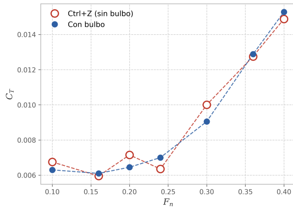
(a) Resistencia total.
