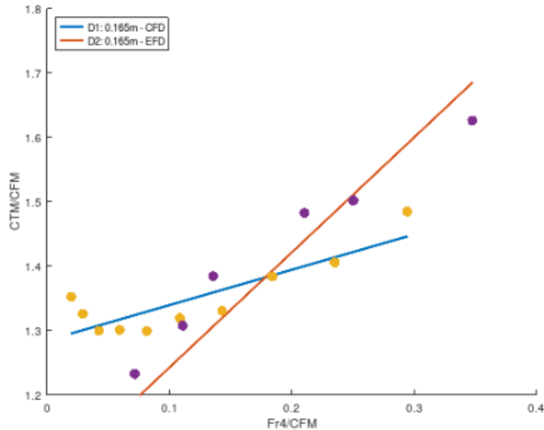
Figura 4.1.16: Diagrama de Prohaska del P1 comparando EFD (D2) y CFD (D1) en función de Fn^4/C_{F0} . Calado 1.
