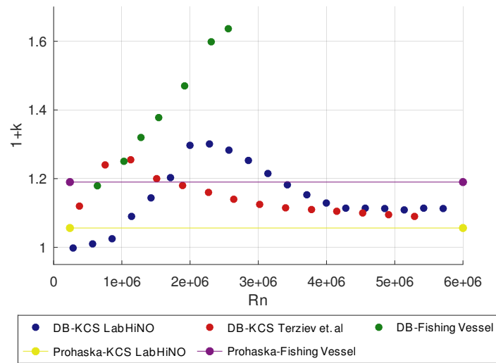
Figura 4.1.21: (1+k) frente a R_n para el KCS (CFD DB, escalas 1:79 y 1:75 de Terziev et al. [2021], y EFD a 1:79) y para el P1 (CFD DB y EFD, escala 1:20, Calado 3).
