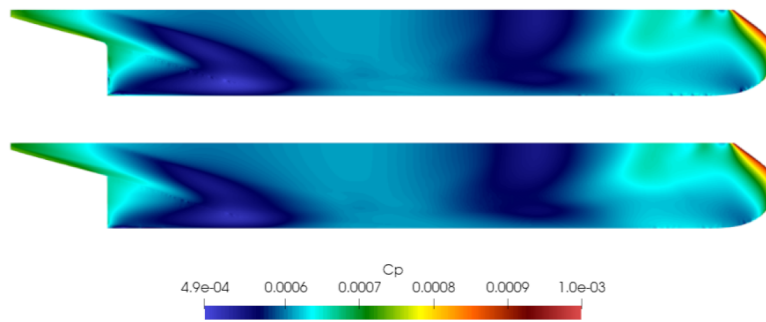
Figura 4.1.32: C_P para F_n = 0,2 , vista lateral. Arriba: escala 1:20. Abajo: escala 1:1.
