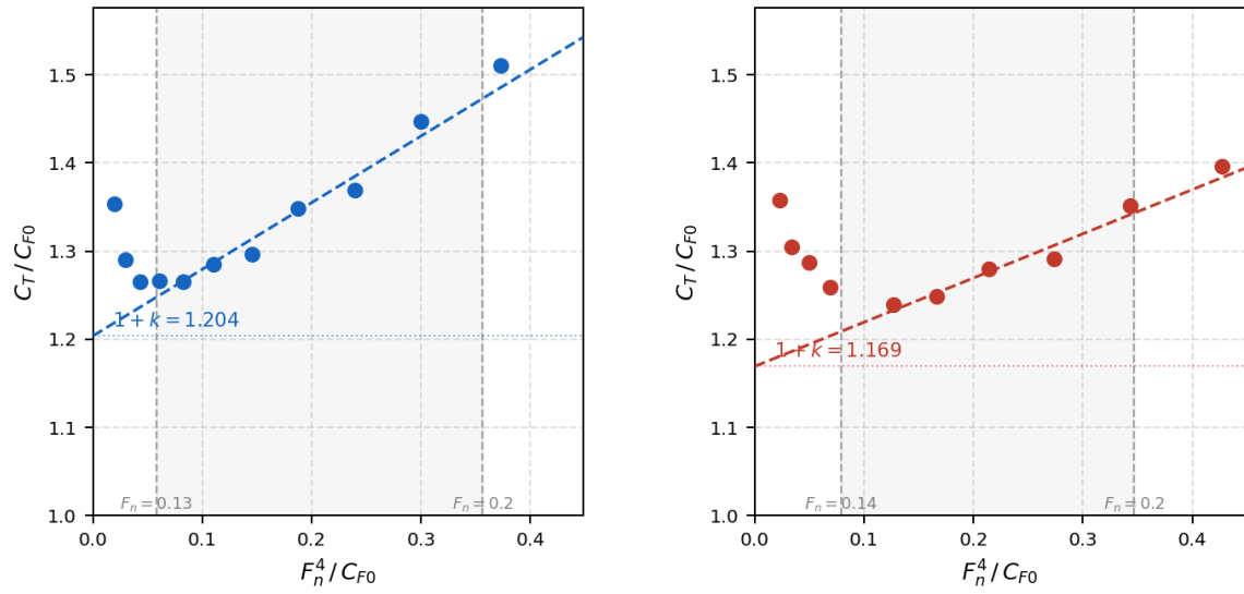
Figura 4.2.2: Diagrama de Prohaska comparando modelos con y sin bulbo ( T = 0,165 m).
