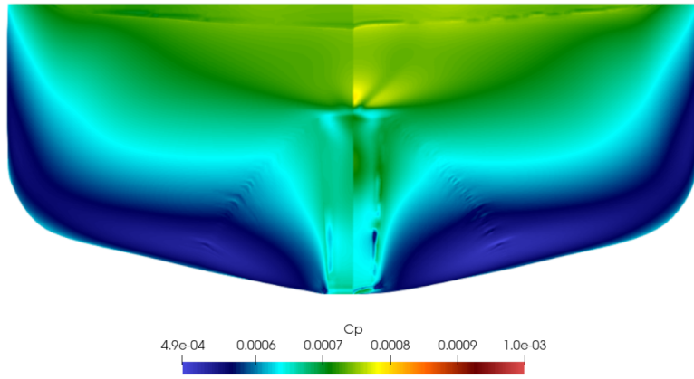
Figura 4.1.30: C_P para F_n = 0,2 , vista de popa. Izquierda: escala 1:20. Derecha: escala 1:1.
