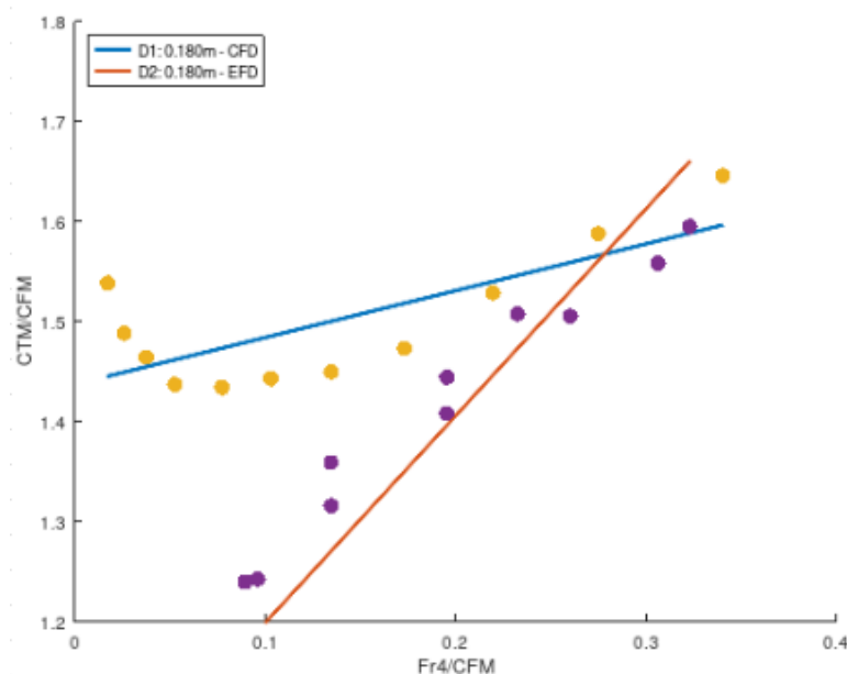
Figura 4.1.17: Diagrama de Prohaska del P1 comparando EFD (D2) y CFD (D1) en función de Fn^4/C_{F0} . Calado 2.
