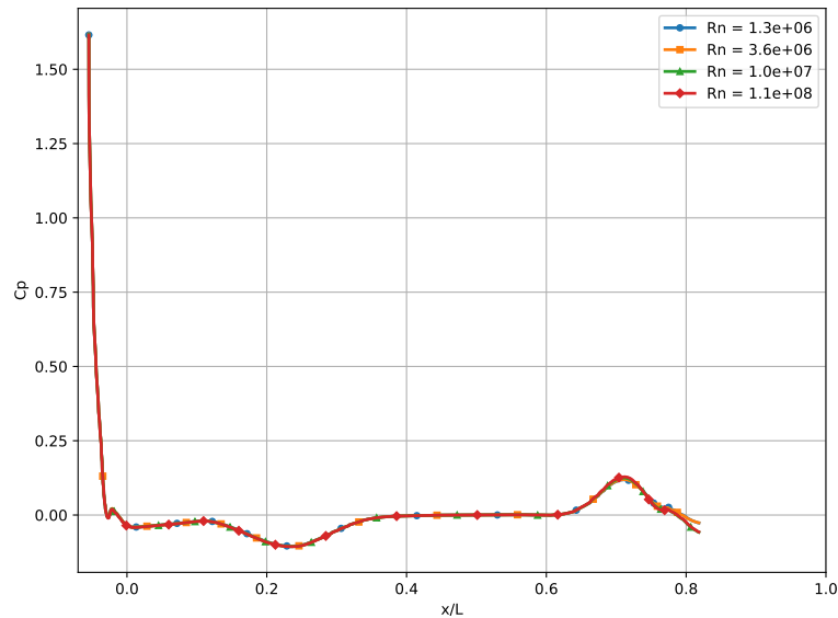
Figura 4.1.34: Distribución de C_P(x/L) sobre el plano z/T = 0,5 .
