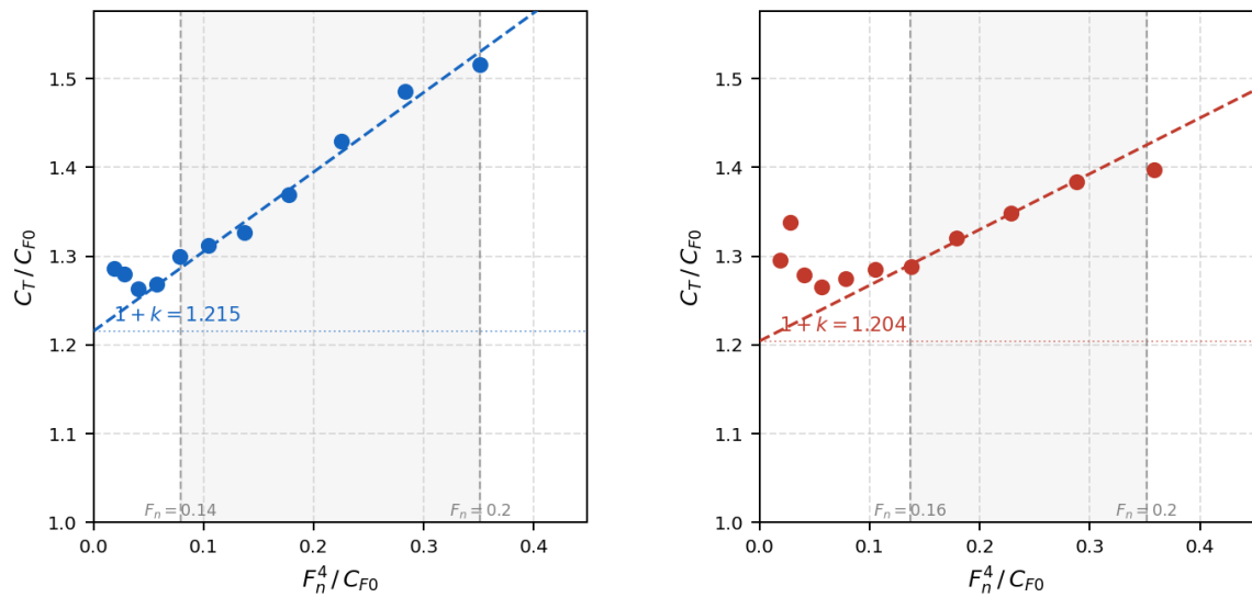
Figura 4.2.3: Diagrama de Prohaska comparando modelos con y sin bulbo ( T = 0,195 m).
