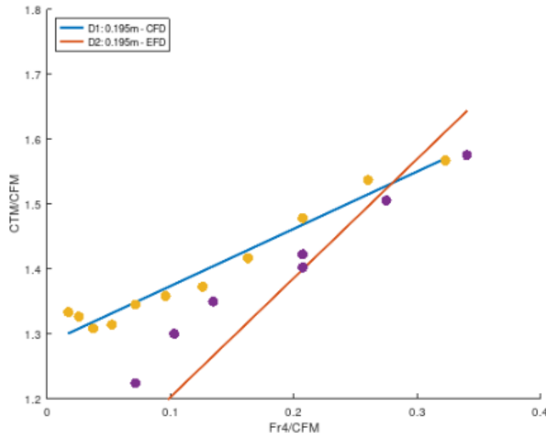
Figura 4.1.18: Diagrama de Prohaska del P1 comparando EFD (D2) y CFD (D1) en función de Fn^4/C_{F0} . Calado 3.
