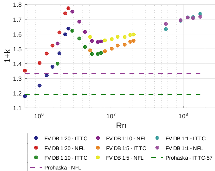
Figura 4.4.1: Variación de (1+k) en función de R_n para el P1 empleando la línea ITTC-57 y la NFL de Korkmaz et al. [2019].
