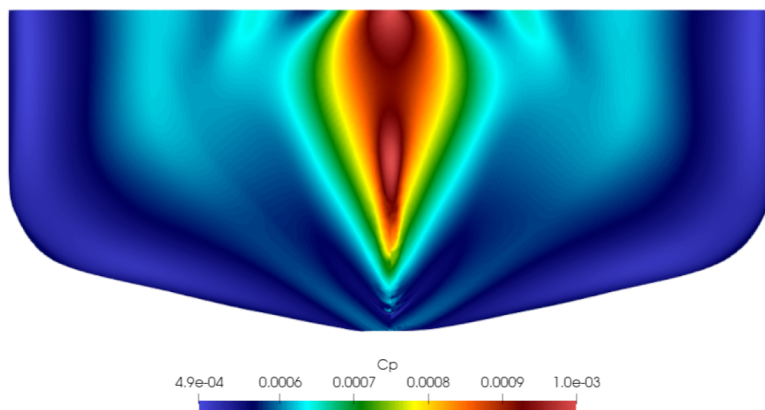
Figura 4.1.29: C_P para F_n = 0,2 , vista de proa. Izquierda: escala 1:20. Derecha: escala 1:1.
