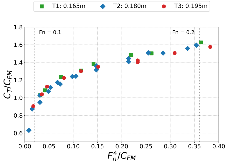
Figura 4.1.2: Diagramas del método de Prohaska para los tres calados del P1 . La desviación respecto de la linealidad teórica se acentúa a bajos números de Froude.
