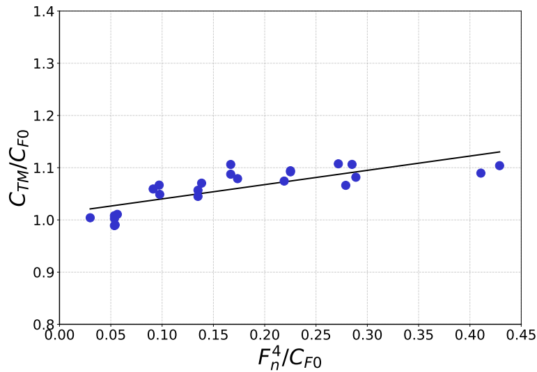
Figura 4.1.5: Diagrama de Prohaska para el modelo KCS. Se grafica C_{TM}/C_{F0} frente a F_n^4/C_{F0} , donde C_{F0} es el coeficiente de fricción de placa plana al Rn del modelo según la línea ITTC-57. La línea continua representa el ajuste por mínimos cuadrados, cuya extrapolación al origen permite obtener el valor de 1 + k .
