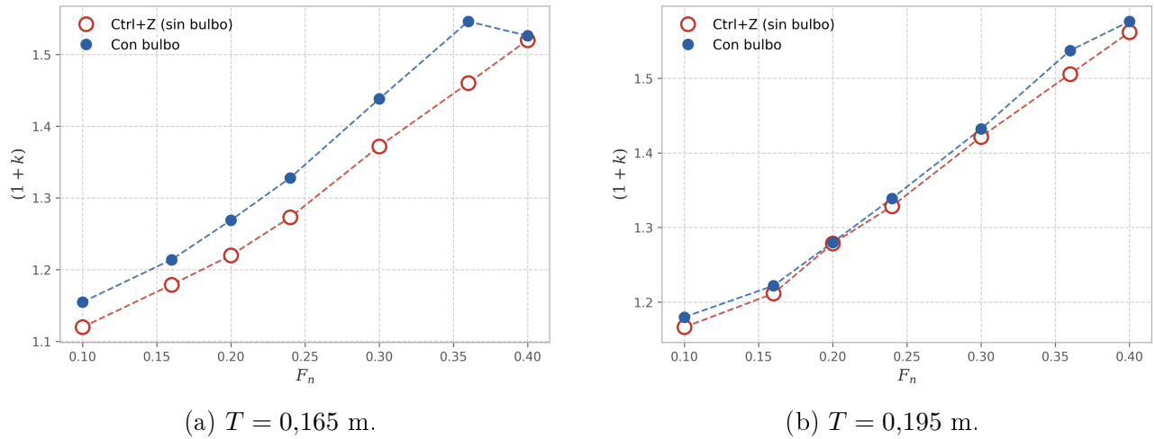
Figura 4.2.6: Factor de forma (1+k) del P1 con y sin proa bulbo en función del número de Froude, para ambos calados.
