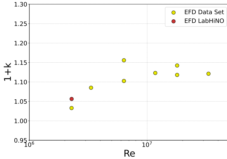
Figura 4.1.7: Comparación del factor de forma ( 1+k ) del KCS obtenido en el LabHiNO (punto rojo) con resultados de distintos laboratorios internacionales recopilados por Terziev et al. [2020] (puntos amarillos), en función del número de Reynolds.
