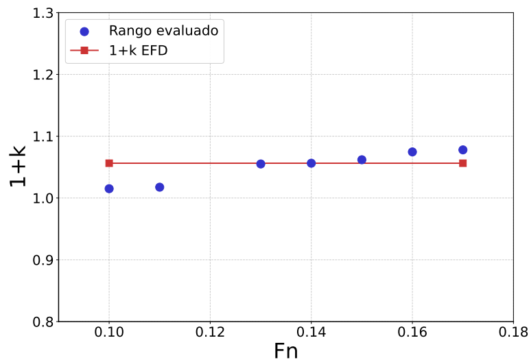
Figura 4.1.6: Variación del factor de forma (1 + k) para el modelo KCS en función del límite inferior del rango de Froude utilizado en el ajuste de Prohaska, con límite superior fijo en F_n = 0,20 . El cuadrado rojo indica el valor adoptado.
