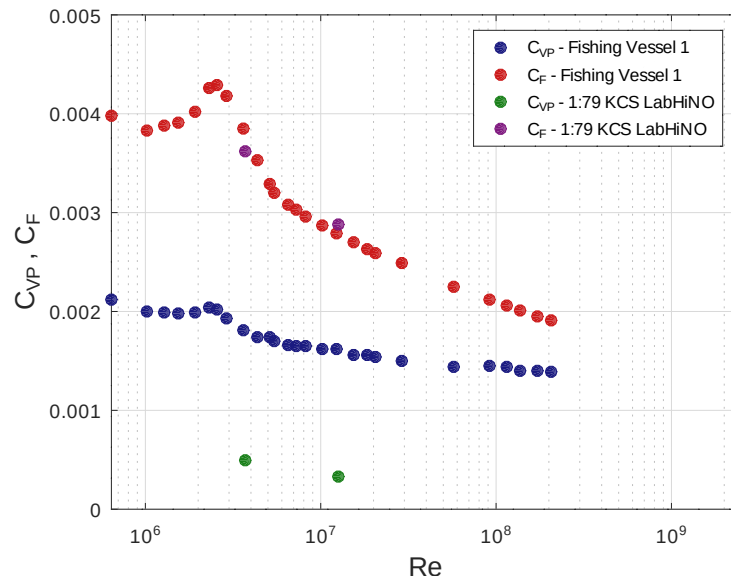
Figura 4.1.26: C_{PV} y C_F obtenidos mediante CFD en doble cuerpo para el P1 y para el KCS 1:79 (LabHiNO).
