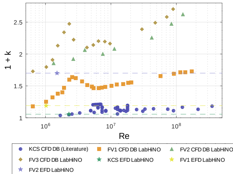
Figura 4.1.23: Evolución de (1+k) con el número de Reynolds para el KCS y los tres pesqueros analizados.
