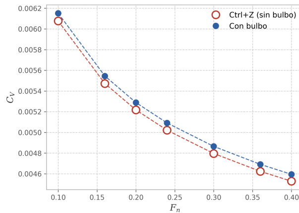
(c) Resistencia viscosa.
