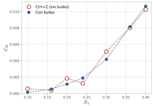
(b) Resistencia por olas.
