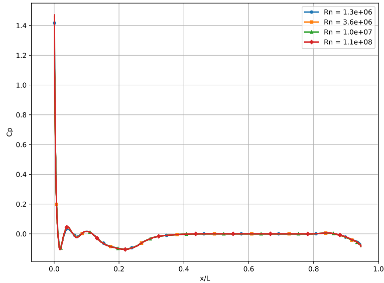
Figura 4.1.33: Distribución de C_P(x/L) sobre el plano z/T = 0 (línea de flotación). Se observa un déficit persistente de presión en popa y variaciones mínimas entre escalas.
