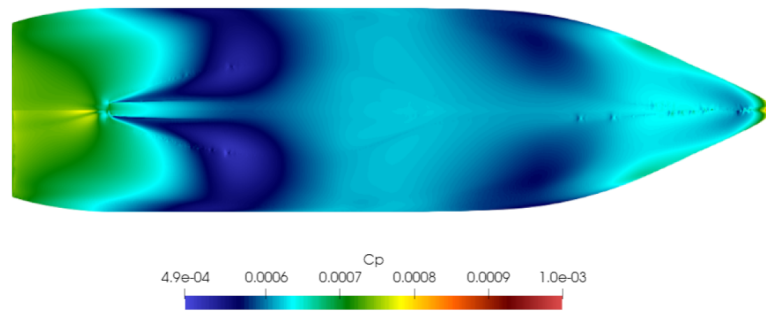
Figura 4.1.31: C_P para F_n = 0,2 , vista desde el fondo. Arriba: escala 1:20. Abajo: escala 1:1.
