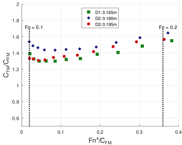
Figura 4.1.10: Diagramas del método de Prohaska para los tres calados del P1 . La desviación respecto de la linealidad teórica se acentúa a bajos números de Froude.
