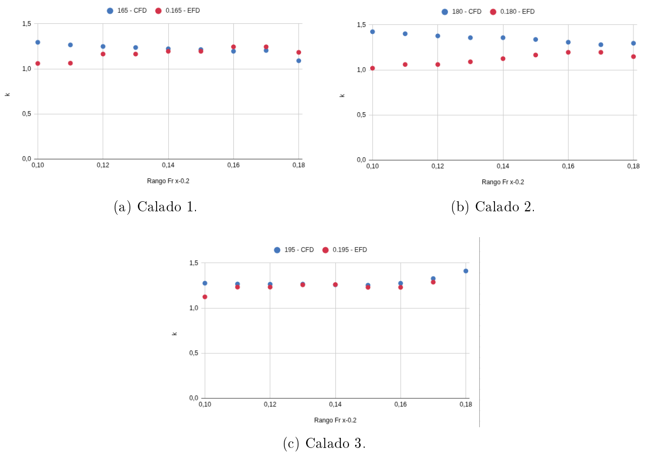
Figura 4.1.19: Variación del factor de forma (1 + k) del P1 , obtenido mediante el método de Prohaska a partir de EFD y CFD, en función del límite inferior del rango de Froude considerado en el ajuste.
