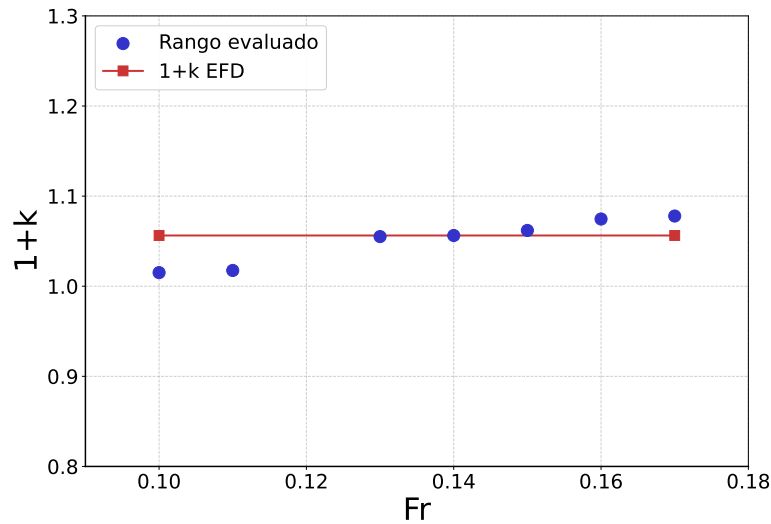
Figura 4.1.7: Variación del factor de forma (1+k) para el modelo KCS en función del límite inferior del rango de Froude utilizado en el ajuste de Prohaska, con límite superior fijo en Fr = 0.20 . El cuadrado rojo indica el valor adoptado.
