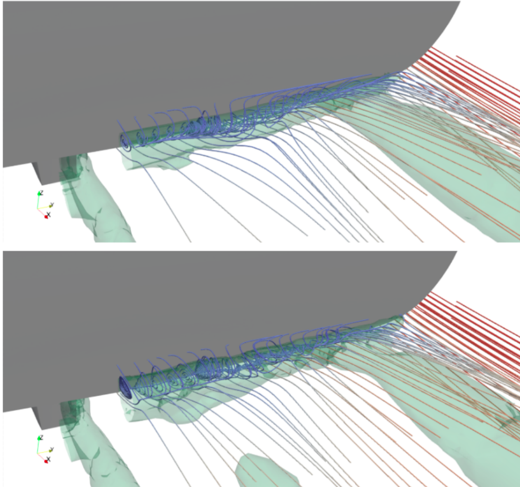
Figura 4.1.29: Iso-superficies de Q-criterio ( Q=10 ) mostrando las estructuras vorticosas presentes en la popa, a escala modelo, 1:20 (arriba, \log(Re) \approx 6 ) y escala buque, 1:1 (abajo, \log(Re) \approx 8 ), a Fr = 0.2 .
