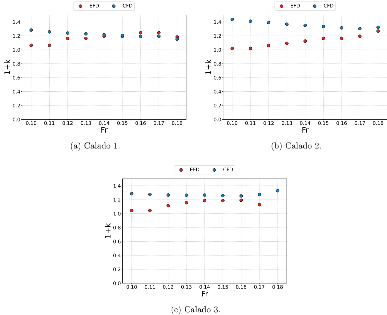
Figura 4.1.20: Variación del factor de forma (1 + k) del P1 , obtenido mediante el método de Prohaska a partir de EFD y CFD, en función del límite inferior del rango de Froude considerado en el ajuste.
