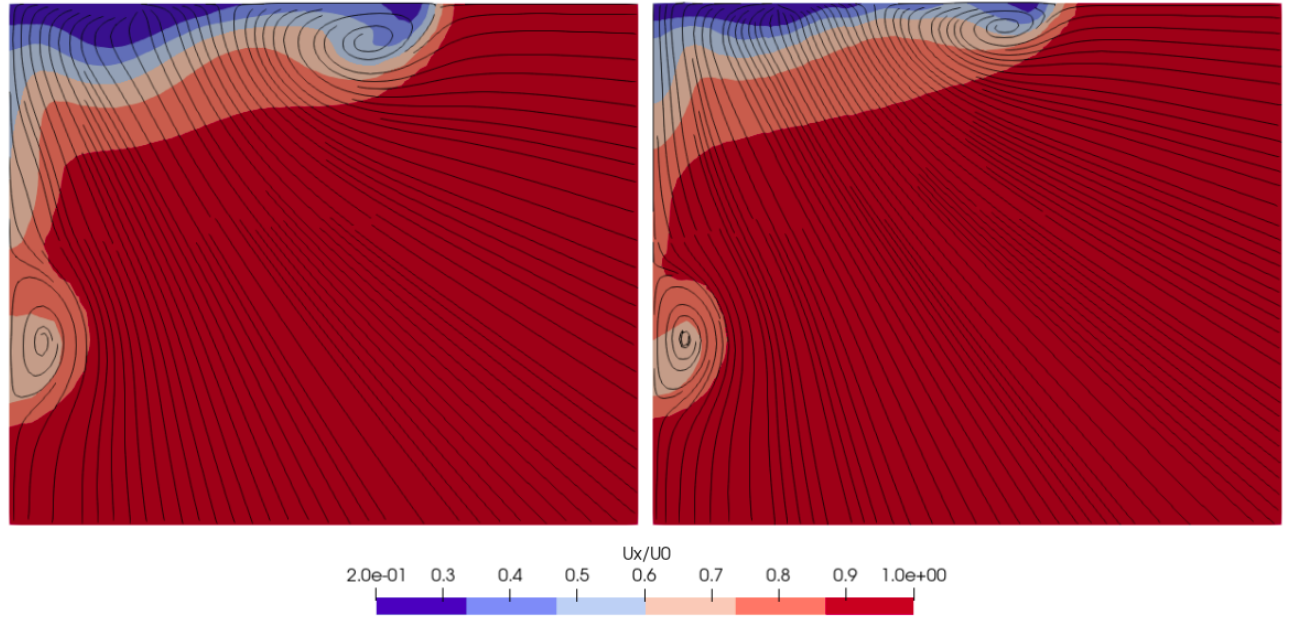
Figura 4.1.28: Contornos de velocidad longitudinal U_x/U_0 en un plano ubicado en x/L = 0.05 para escala modelo, 1:20 (izquierda, \log(Re) \approx 6 ) y escala buque, 1:1 (derecha, \log(Re) \approx 8 ), a Fr = 0.2 .
