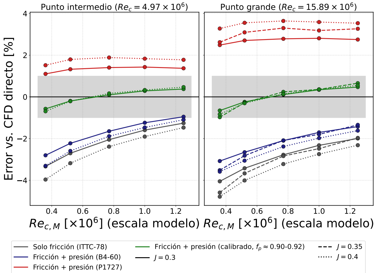
Figura 5.4.2: Error de la extrapolación Fully Turbulent respecto de los dos puntos de validación, para las tres correcciones evaluadas y los tres J calculados.
