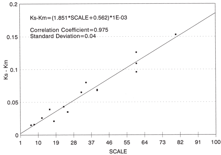
Figura 2.1.2: Efecto de escala del factor de forma, K_S - K_M , en función de la razón de escala \lambda para quince modelos de cuatro familias de geosims, con la recta de regresión de García-Gómez [2000] .
