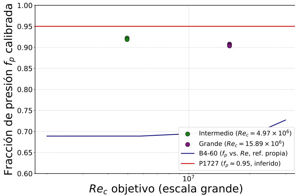
Figura 5.4.1: Fracción de presión calibrada en los dos puntos de escala independientes, comparada con la curva propia de la B4-60 (evaluada en función de Re ) y con el valor inferido del P1727.
