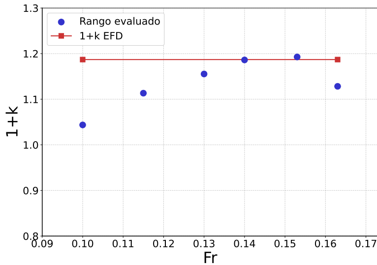
Figura 4.1.3: Variación del factor de forma (1+k) al modificar el límite inferior del rango de Froude (puntos azules), manteniendo el superior en Fr = 0.20 . La línea roja indica el valor de (1+k) adoptado mediante el método de Prohaska en el rango 0.15 < Fr < 0.20 . Calado 3. Comportamiento análogo en otros calados.
