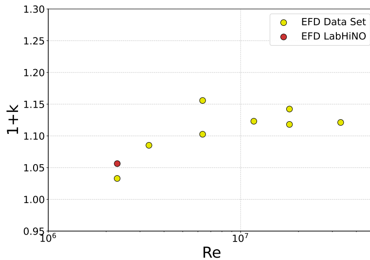
Figura 4.1.8: Comparación del factor de forma (1+k) del KCS obtenido en el LabHiNO (punto rojo) con resultados experimentales históricos del KCS compilados de literatura internacional en Terziev et al. [2020] (puntos amarillos), en función del número de Reynolds.
