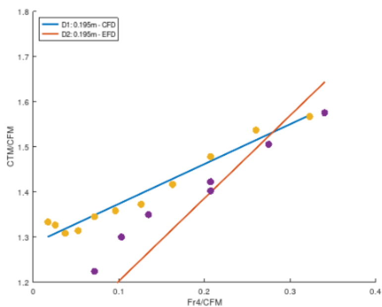
Figura 4.1.16: Resistencia al avance en función de Fr. Calado 1.
