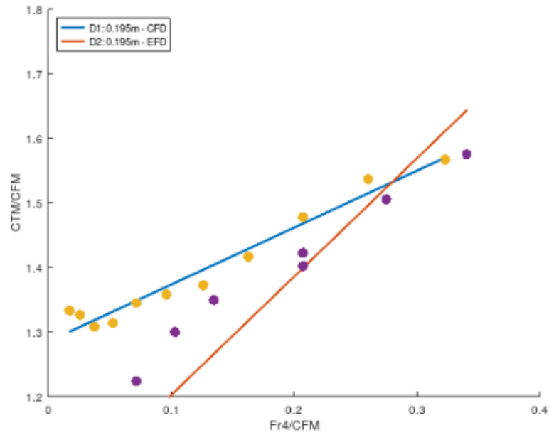
Figura 4.1.17: Resistencia al avance en función de Fr. Calado 2.
