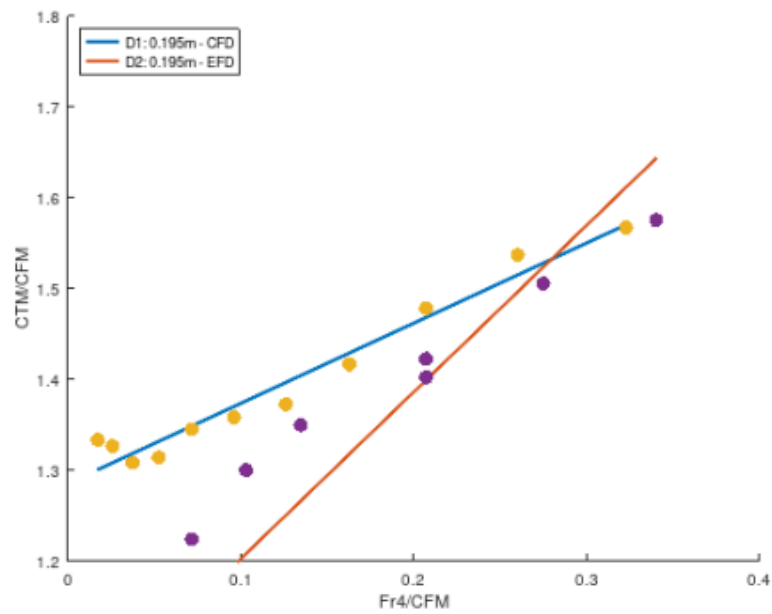
Figura 4.1.18: Resistencia al avance en función de Fr. Calado 3.
