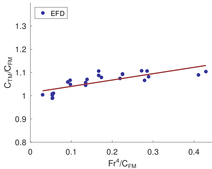
Figura 4.1.9: Determinación experimental del factor de forma (1 + k) para el modelo KCS mediante el método de Prohaska.
