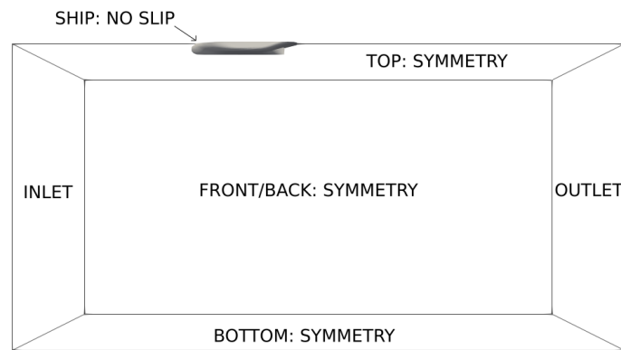
Figura 4.1.19: Dominio reducido para simulación sin superficie libre.
