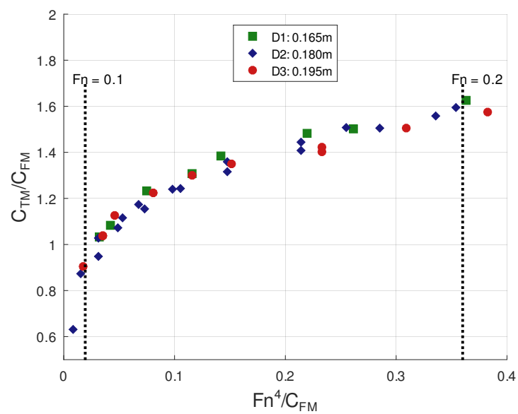
Figura 4.1.4: Diagramas del método de Prohaska para los tres calados del pesquero TPA. La desviación respecto de la linealidad teórica se acentúa a bajos números de Froude.
