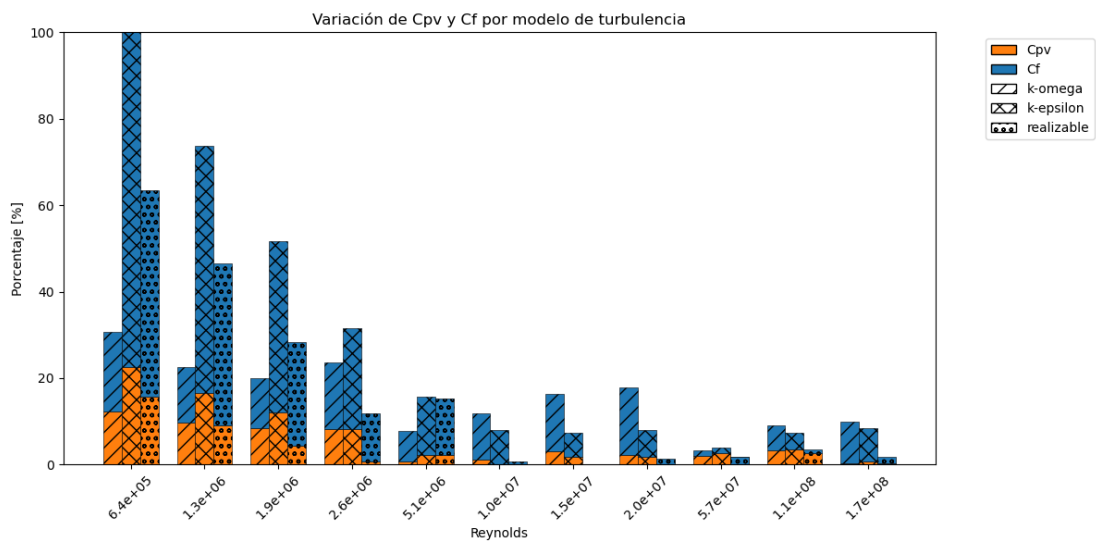
Figura 4.2.19: Diferencia en puntos porcentuales de C_F y C_{PV} respecto al modelo k-ω SST.
