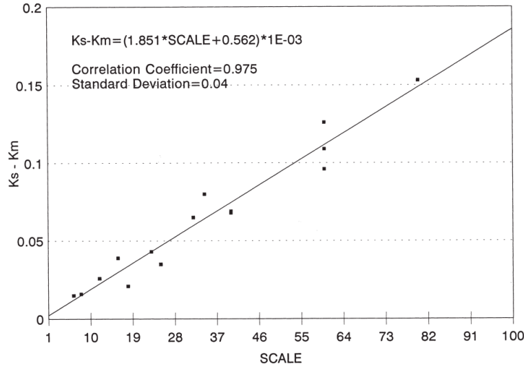
Figura 2.1.2: Efecto de escala del factor de forma, K_S - K_M , en función de la razón de escala \lambda para quince modelos de cuatro familias de geosims, con la recta de regresión de Garcia-Gómez [2000] .
