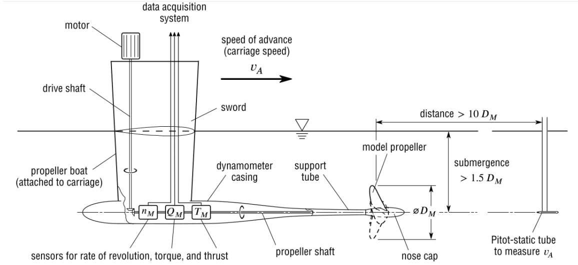
Figura 3.2.8: Esquema del ensayo de aguas abiertas: la hélice, montada sobre el eje portahélice accionado por el dinamómetro de aguas abiertas, opera en flujo uniforme sin casco mientras el carro impone la velocidad de avance V_a y se mide el empuje T y el par Q . Adaptado de Birk [2019].
