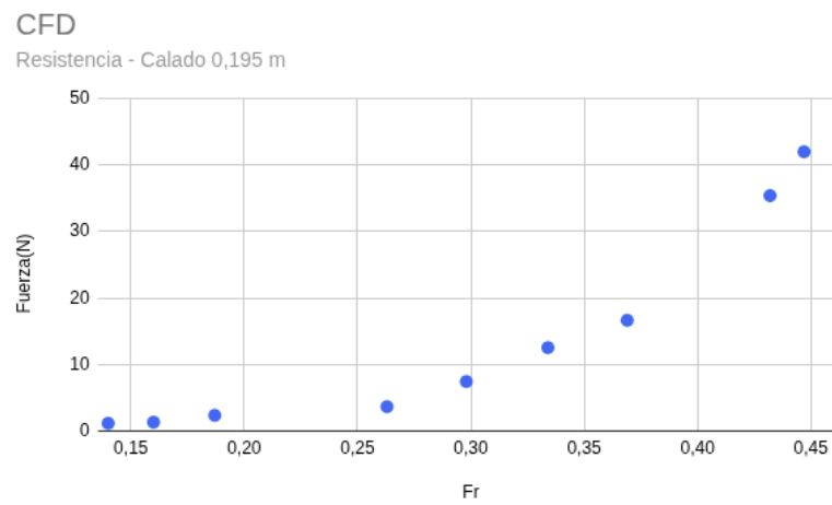
Figura 4.1.14: Resistencia al avance en función de Fr. Calado 3.
