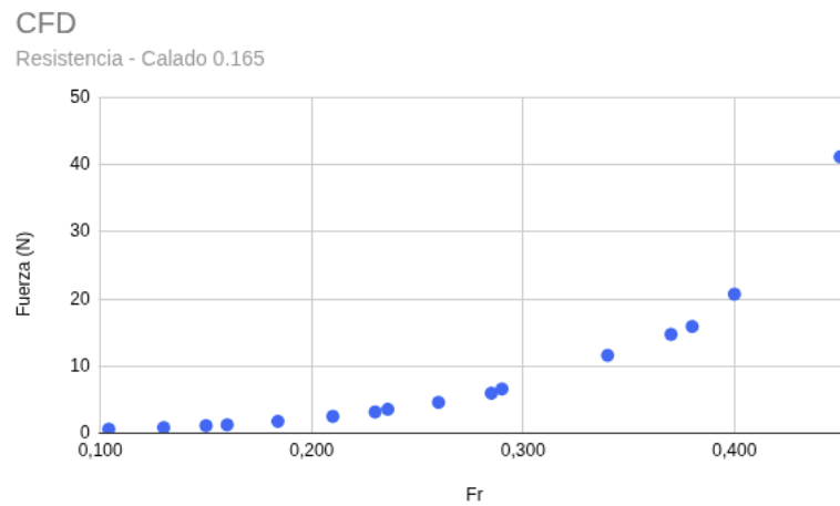
Figura 4.1.13: Resistencia al avance en función de Fr. Calado 2.
