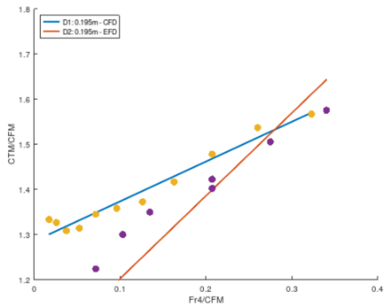
Figura 4.1.17: Resistencia al avance en función de Fr. Calado 3.
