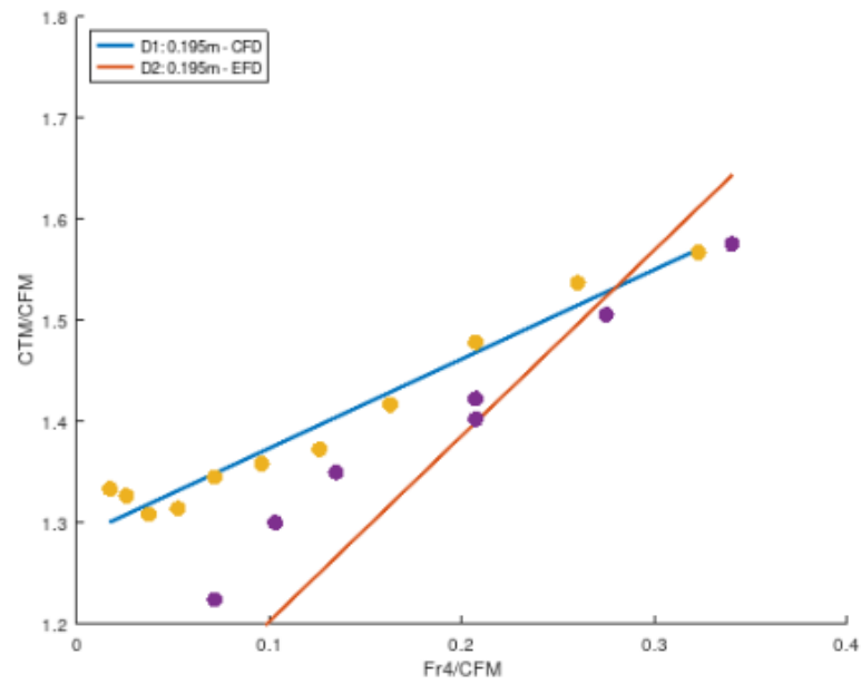
Figura 4.1.16: Resistencia al avance en función de Fr. Calado 2.
