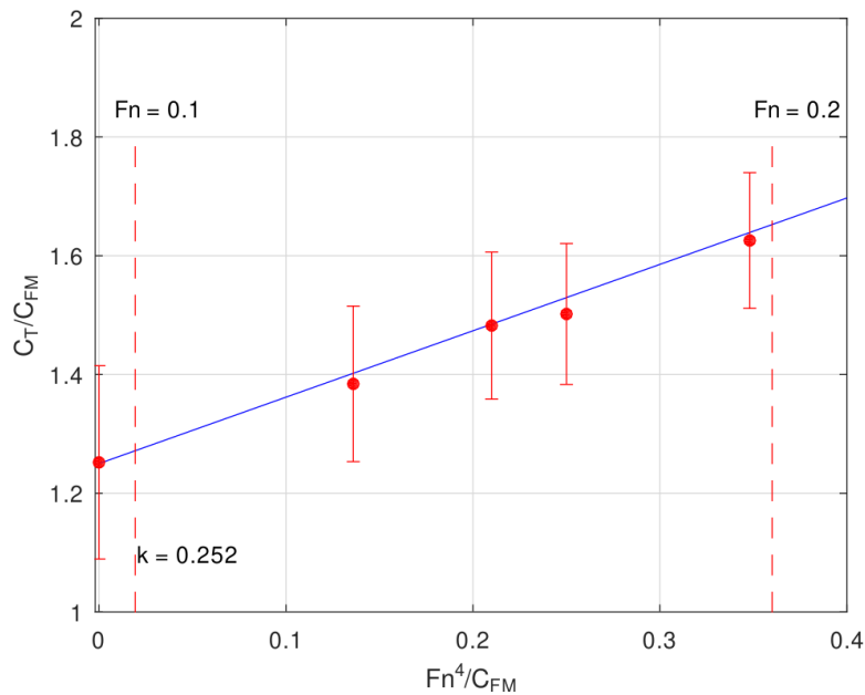
Figura 4.1.7: Ajuste lineal con ponderación mediante el método de York aplicado al pesquero TPA para la estimación de (1 + k) y su incertidumbre.
