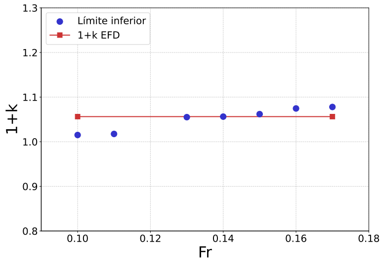
Figura 4.1.8: Variación del factor de forma (1 + k) para el modelo KCS en función del límite inferior del rango de Froude utilizado en el ajuste de Prohaska, con límite superior fijo en Fr = 0.20 . El cuadrado rojo indica el valor adoptado.
