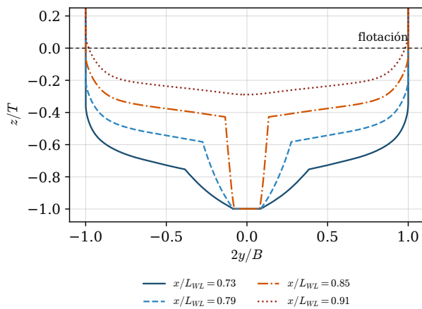
(b) Cuadernas de popa del P1 .
