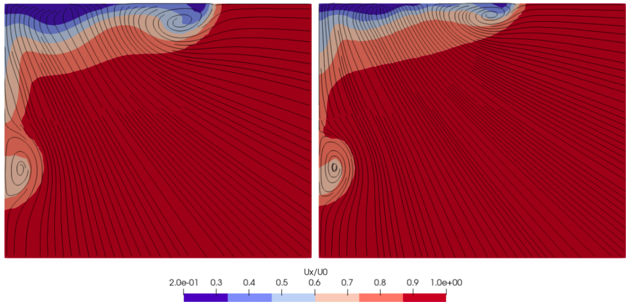
Figura 4.1.39: Contornos de velocidad longitudinal U_x/U_0 en un plano transversal ubicado a 0.05 L_{WL} aguas abajo del espejo, para escala modelo, 1:20 (izquierda, \log(Re) \approx 6 ) y escala buque, 1:1 (derecha, \log(Re) \approx 8 ), a Fr = 0.2 y calado 0.195 m (T3). En cada panel, el borde izquierdo corresponde al plano de crujía y la parte superior se ubica hacia la superficie libre. Foco inferior: vórtice de quilla; foco superior: vórtice de pantoque.
