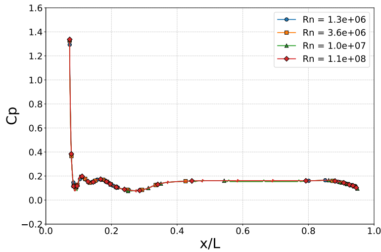
Figura 4.1.45: Distribución de C_P(x/L) sobre el plano |z|/T = 0 (línea de flotación). Se observa un déficit persistente de presión en popa y variaciones mínimas entre escalas.
