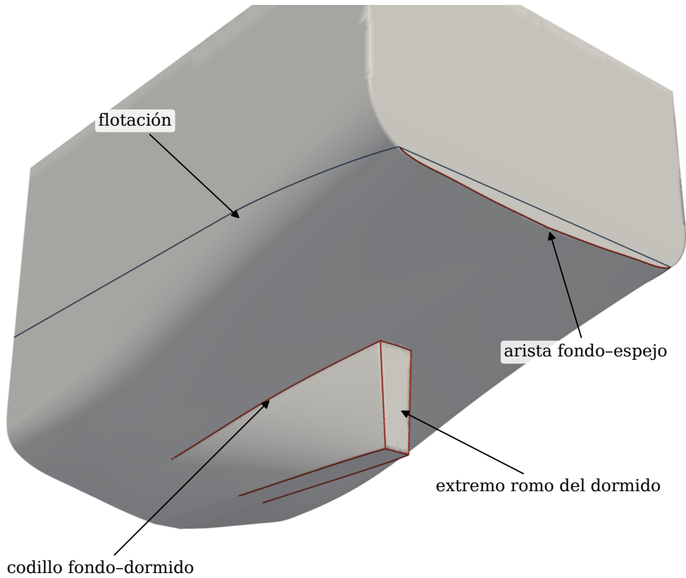
(a) Popa del P1 ; en rojo, aristas vivas sumergidas, identificadas como bordes con un cambio de orientación entre caras superior a 20^\circ ; en azul, línea de flotación.
