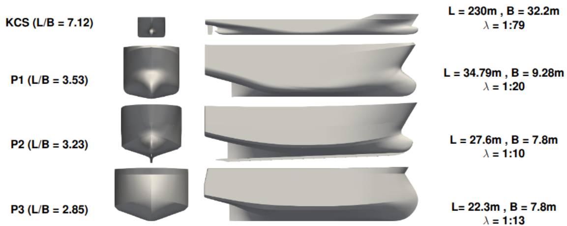
Figura 4.6.4: Modelos ensayados. Los cuatro cascos son presentados con la misma eslora para comparación directa de su esbeltez.
