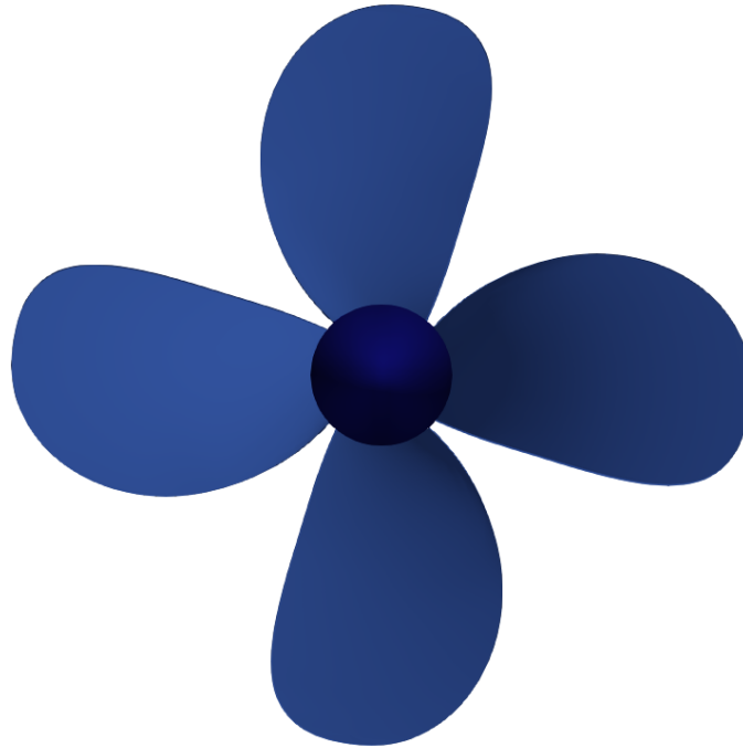
Figura 3.2.6: Geometría de la hélice de referencia Wageningen B4-60.
