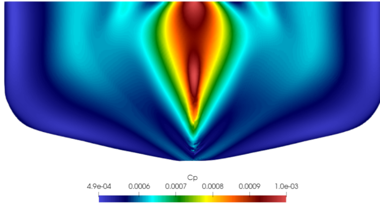
Figura 4.1.41: C_P para Fr = 0.2 , vista de proa. Izquierda: escala 1:20. Derecha: escala 1:1.
