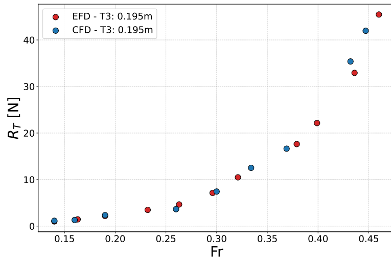
Figura 4.1.22: Resistencia al avance del P1 en función de Fr . Comparación EFD–CFD para el Calado 0.195 m (T3).
