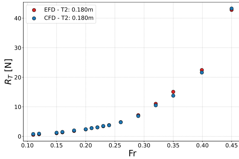
Figura 4.1.21: Resistencia al avance del P1 en función de Fr . Comparación EFD–CFD para el Calado 0.180 m (T2).
