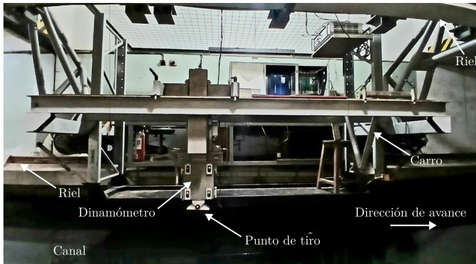
Figura 3.2.5: Montaje del ensayo de resistencia.
