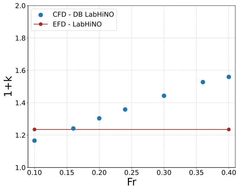
Figura 4.1.29: Comparación entre el valor de (1 + k) adoptado por Prohaska EFD (línea horizontal roja) y los valores obtenidos mediante el método de doble cuerpo (DB) en función de Fr (puntos azules) para el P1 , Calado 1.
