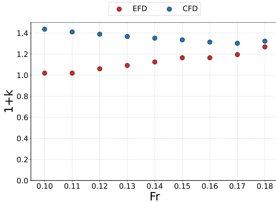
Figura 4.1.27: Variación del factor de forma (1+k) del P1 para el Calado 0.180 m (T2), obtenido mediante el método de Prohaska a partir de EFD y CFD, en función del límite inferior del rango de Froude considerado en el ajuste.
