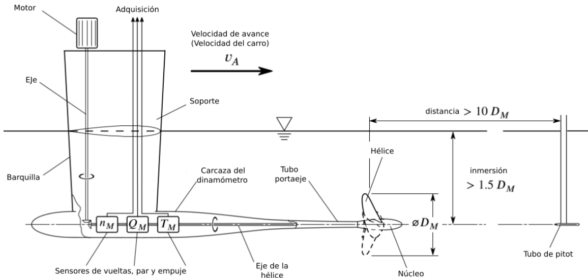
Figura 3.2.8: Esquema del ensayo de aguas abiertas en canal. Adaptado de Birk (2019).
