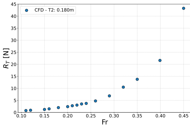
Figura 4.1.13: Resistencia total al avance del P1 obtenida por CFD en función de Fr para el Calado 0.180 m (T2).
