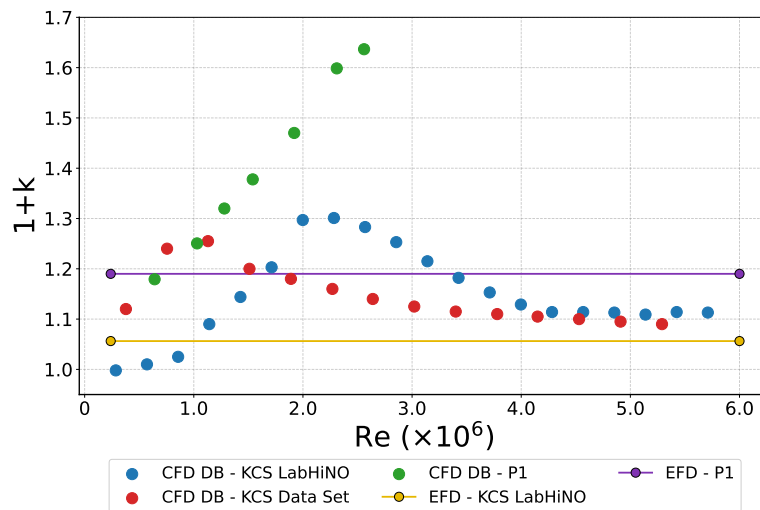
Figura 4.1.32: (1+k) frente a Re para el KCS (CFD DB, escalas 1:79 y 1:75 de Terziev et al. (2021), y EFD a 1:79) y para el P1 (CFD DB y EFD, escala 1:20, calado 0.195 m, T3).
