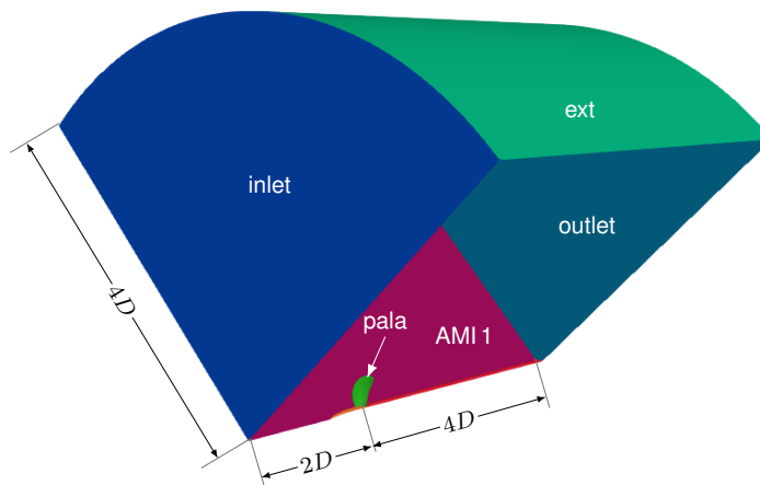
Figura 3.4.3: Dominio computacional empleado en las simulaciones (sector de 90^\circ con interfaz periódica AMI). Las distancias se expresan en diámetros de hélice D .
