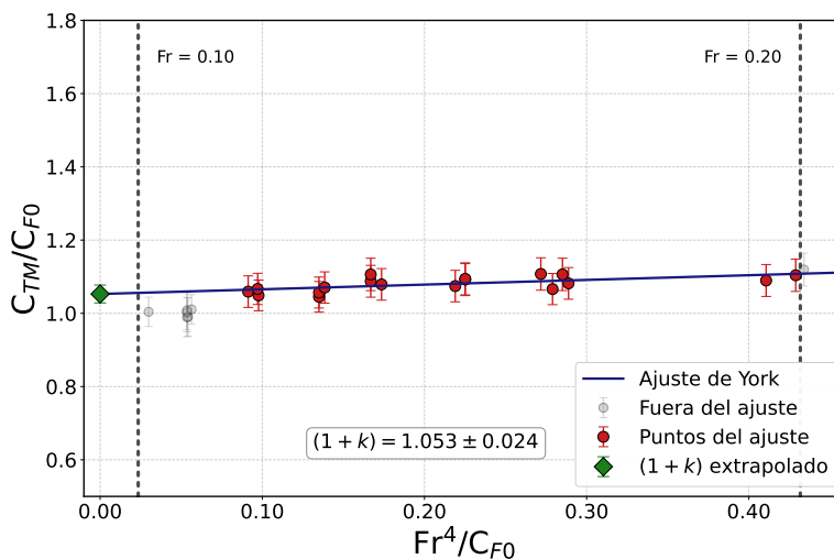
Figura 4.1.9: Ajuste lineal con ponderación mediante el método de York aplicado al KCS para la estimación de (1 + k) y su incertidumbre. Las líneas verticales punteadas indican Fr = 0.10 y Fr = 0.20 para el KCS .
