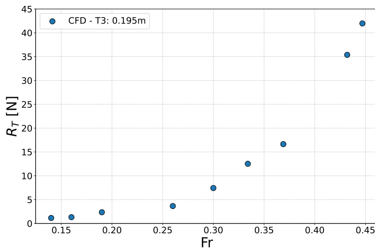
Figura 4.1.14: Resistencia total al avance del P1 obtenida por CFD en función de Fr para el Calado 0.195 m (T3).
