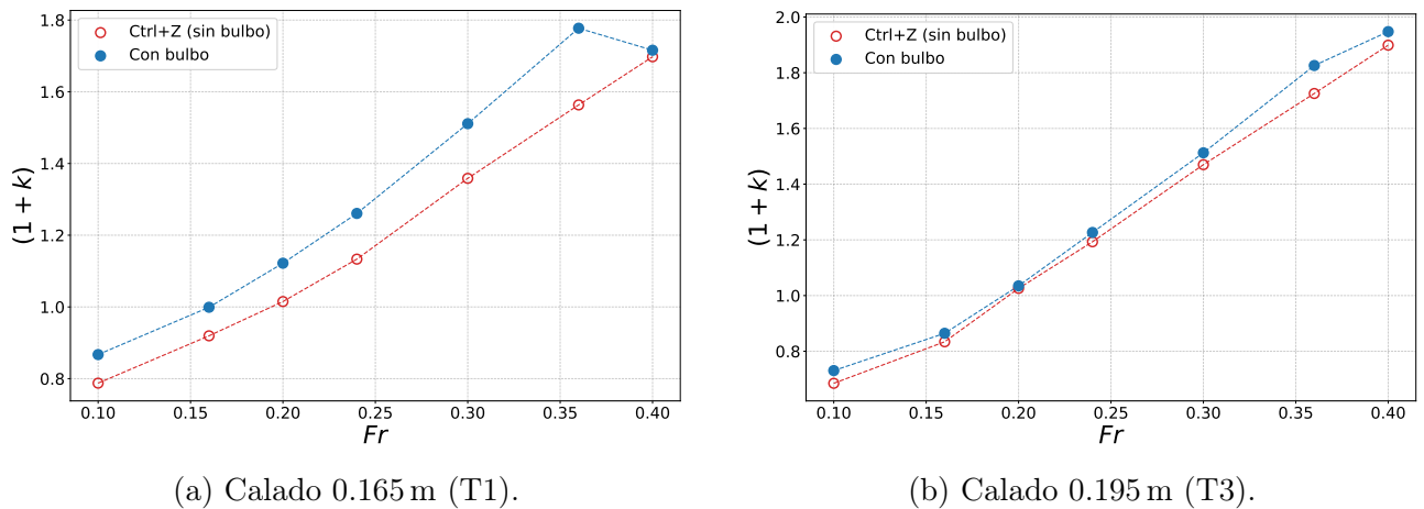
Figura 4.2.4: Factor de forma (1 + k) del P1 con y sin proa bulbo, obtenido mediante el método de doble cuerpo (DB), en función del número de Froude, para ambos calados.
