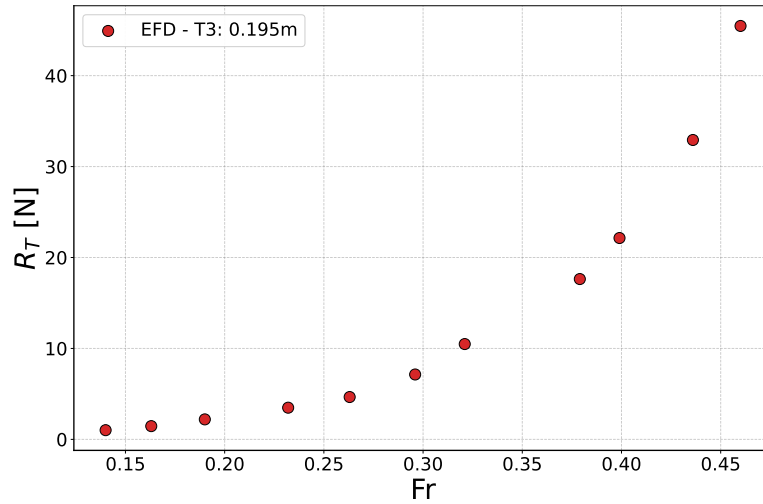
Figura 4.1.3: Resistencia total al avance (EFD) en función de Fr para el Calado 0.195 m (T3).
