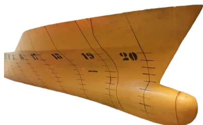
(a) Vista en perspectiva de proa. Se observan las marcas de calado y los estimuladores de turbulencia.
