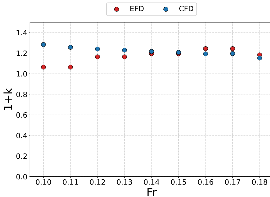
Figura 4.1.26: Variación del factor de forma (1+k) del P1 para el Calado 0.165 m (T1), obtenido mediante el método de Prohaska a partir de EFD y CFD, en función del límite inferior del rango de Froude considerado en el ajuste.
