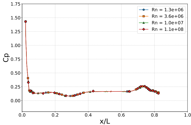
Figura 4.1.46: Distribución de C_P(x/L) sobre el plano |z|/T = 0.5 .
