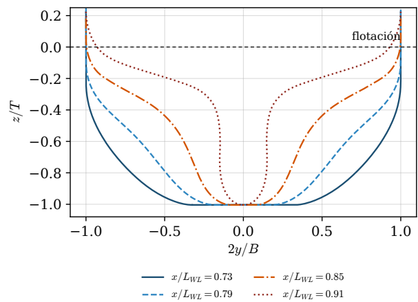
(c) Cuadernas de popa del KCS .
