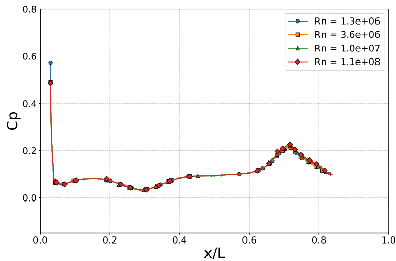
Figura 4.1.47: Distribución de C_P(x/L) sobre el plano |z|/T = 0.75 .
