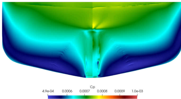
Figura 4.1.42: C_P para Fr = 0.2 , vista de popa. Izquierda: escala 1:20. Derecha: escala 1:1.
