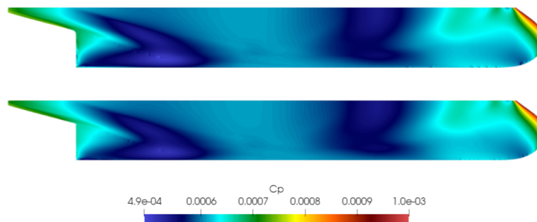
Figura 4.1.44: C_P para Fr = 0.2 , vista lateral. Arriba: escala 1:20. Abajo: escala 1:1.
