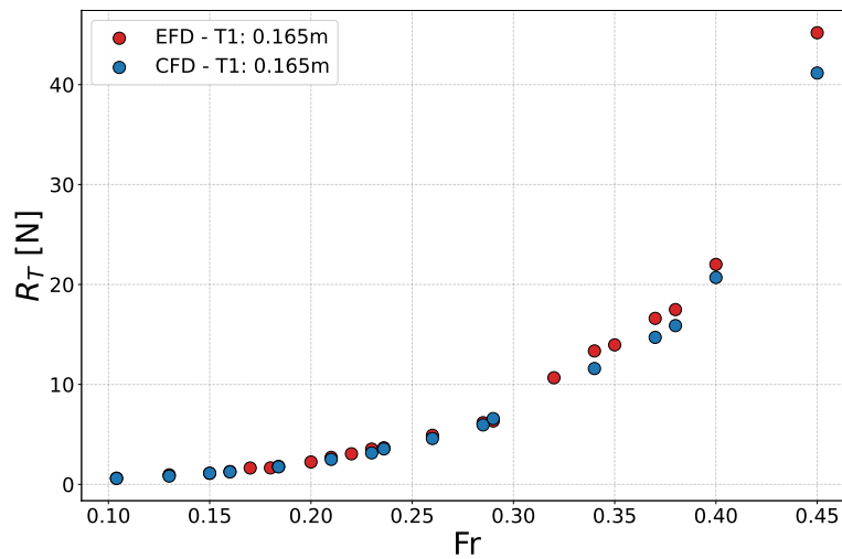
Figura 4.1.20: Resistencia al avance del P1 en función de Fr . Comparación EFD–CFD para el Calado 0.165 m (T1).
