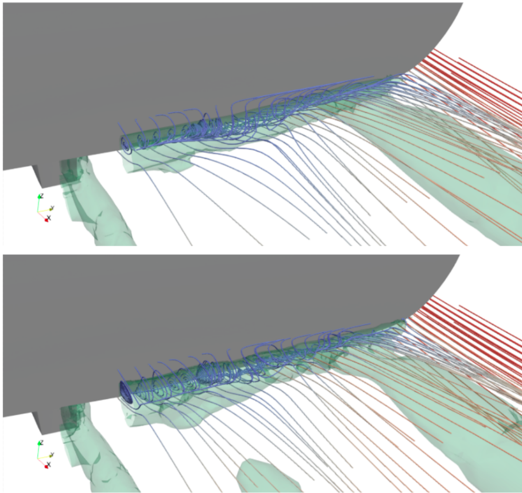
Figura 4.1.40: Iso-superficies del criterio Q ( Q = 10 , en verde) y líneas de corriente en la popa del P1 , a escala modelo, 1:20 (arriba, \log(Re) \approx 6 ) y escala buque, 1:1 (abajo, \log(Re) \approx 8 ), a Fr = 0.2 .
