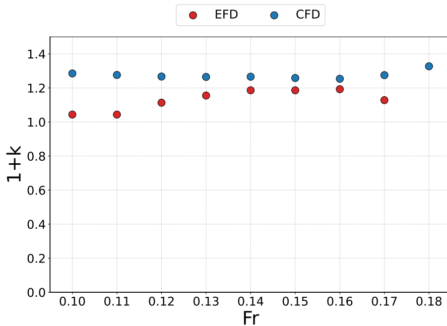
Figura 4.1.28: Variación del factor de forma (1+k) del P1 para el Calado 0.195 m (T3), obtenido mediante el método de Prohaska a partir de EFD y CFD, en función del límite inferior del rango de Froude considerado en el ajuste.
