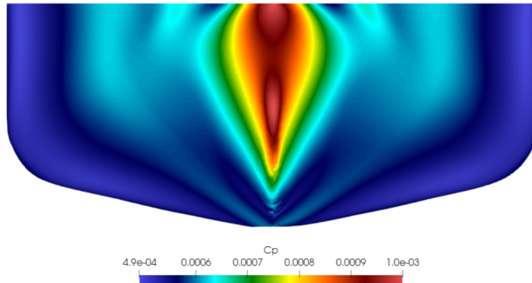
Figura 4.1.29: C_P para F_n = 0,2 , vista de proa. Izquierda: escala 1:20. Derecha: escala 1:1.
