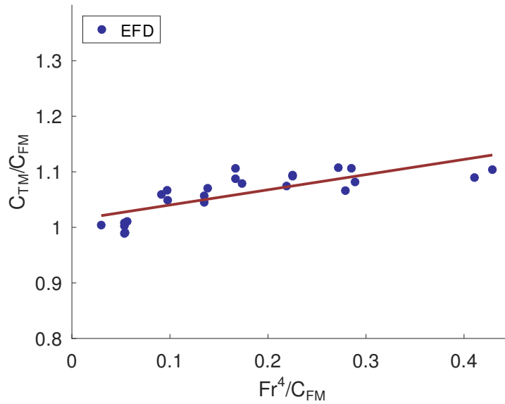
Figura 4.1.5: Diagrama de Prohaska para el modelo KCS. Se grafica C_{TM}/C_{F0} frente a Fn^4/C_{F0} , donde C_{F0} es el coeficiente de fricción de placa plana al Rn del modelo según la línea ITTC-57. La recta de regresión se obtuvo mediante el método de York [York et al., 2004].
