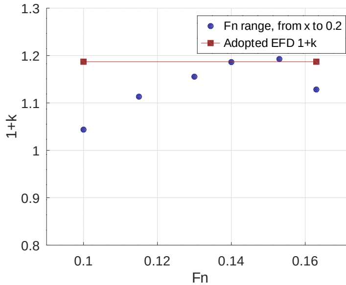
Figura 4.1.3: Variación del factor de forma experimental ( 1+k ) para el P1 en función del límite inferior del rango de Froude utilizado en el ajuste de Prohaska, con límite superior fijo en F_n = 0,20 . El cuadrado rojo indica el valor adoptado. Calado 3; los demás calados presentaron comportamiento análogo.
