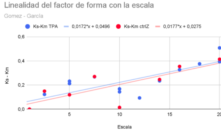
Figura 4.1.24: Linealidad del factor de forma con la escala para el P1 , siguiendo el método de García-Gómez [2000].
