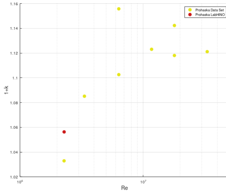
Figura 4.1.7: Comparación del factor de forma ( 1 + k ) del KCS obtenido en el LabHiNO (punto rojo) con resultados de distintos laboratorios internacionales recopilados por Terziev et al. [2020] (puntos amarillos), en función del número de Reynolds.
