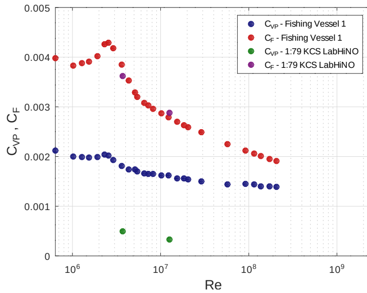
Figura 4.1.26: C_{PV} y C_F obtenidos mediante CFD en doble cuerpo para el P1 y para el KCS 1:79 (LabHiNO).
