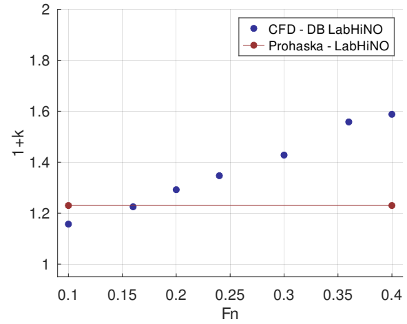
(b) Calado 2.
