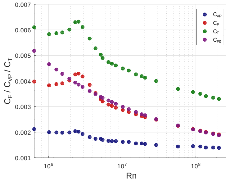
Figura 4.1.25: Coeficientes C_T , C_{PV} y C_F obtenidos mediante CFD en configuración de doble cuerpo, junto con la línea ITTC-57 ( C_{F0} ), en función de R_n para el P1 .
