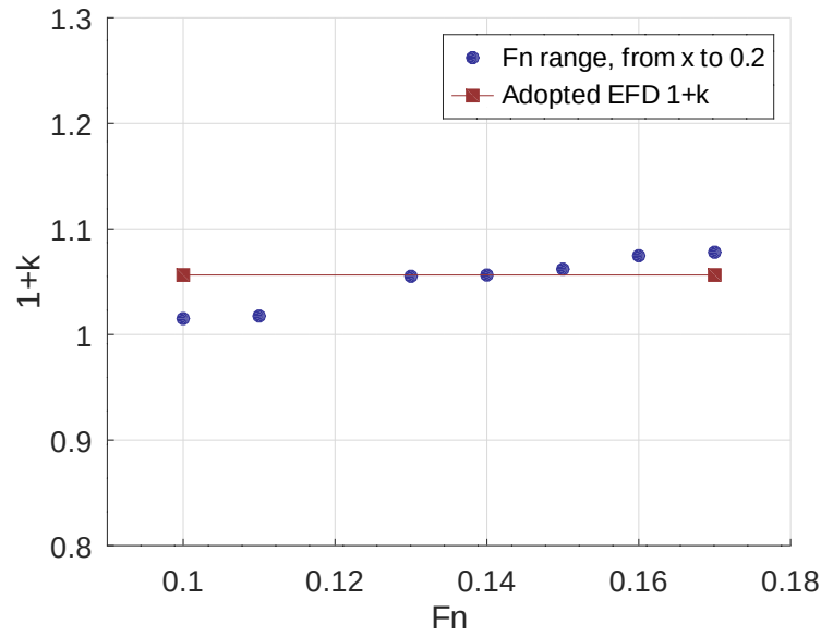
Figura 4.1.6: Variación del factor de forma ( 1 + k ) para el modelo KCS en función del límite inferior del rango de Froude utilizado en el ajuste de Prohaska, con límite superior fijo en F_n = 0,20 . El cuadrado rojo indica el valor adoptado.
