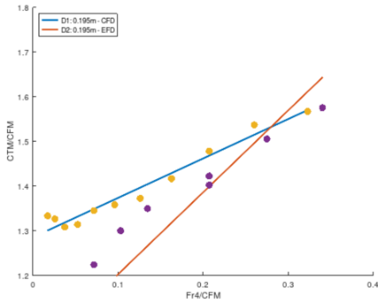
Figura 4.1.18: Diagrama de Prohaska del P1 comparando EFD (D2) y CFD (D1) en función de Fn^4/C_{F0} . Calado 3.
