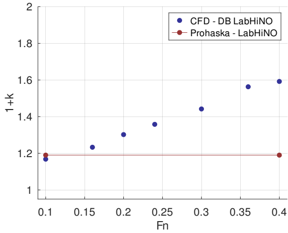
(a) Calado 1.
