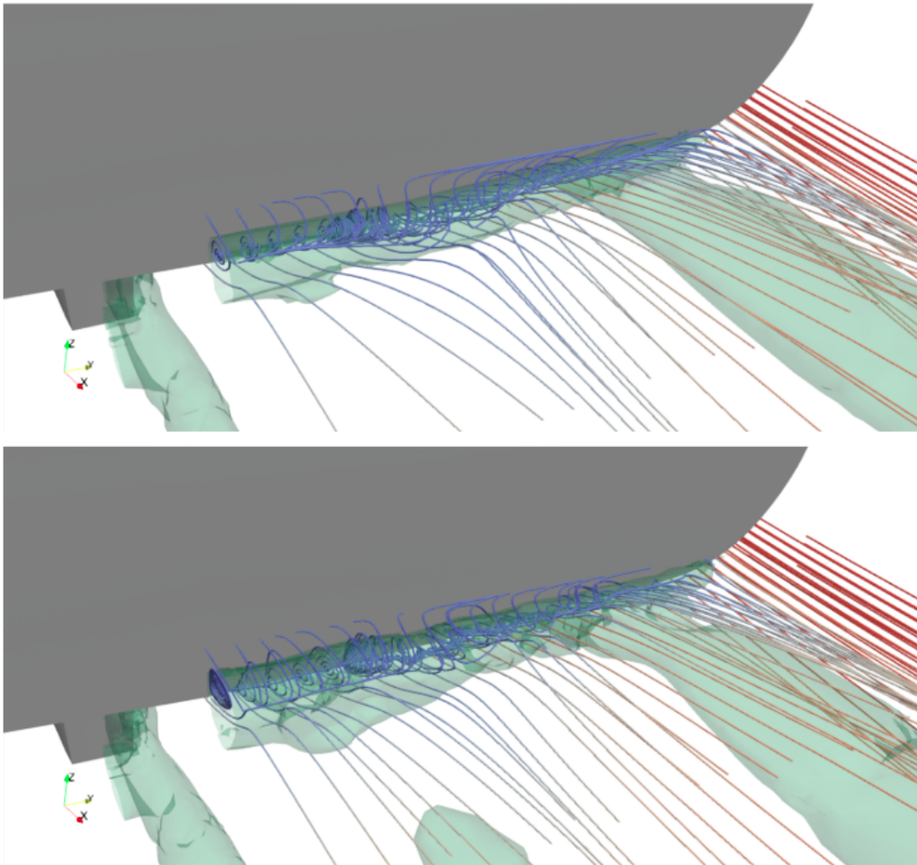
Figura 4.1.28: Iso-superficies de Q-criterio ( Q=10 ) mostrando las estructuras vorticosas presentes en la popa, a escala modelo, 1:20 (arriba, \log(Re) \approx 6 ) y escala buque, 1:1 (abajo, \log(Re) \approx 8 ), a Fr = 0,2 .
