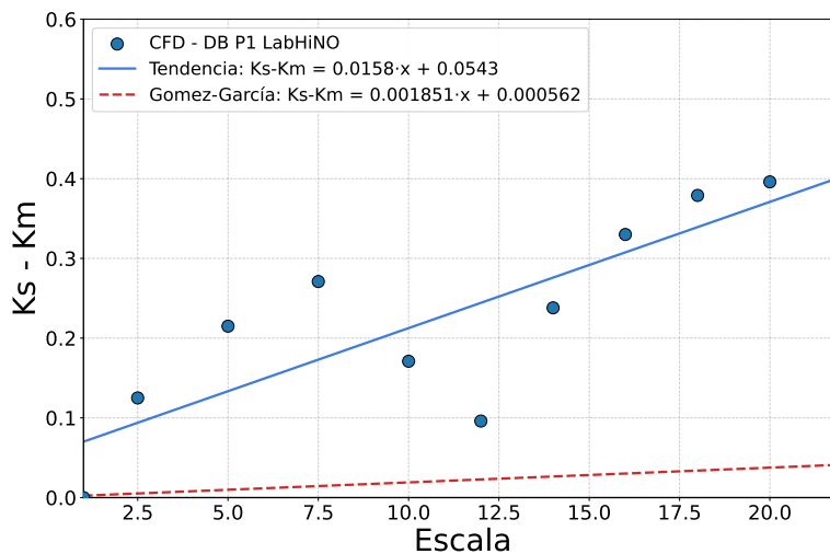
Figura 4.1.24: Linealidad del factor de forma con la escala para el P1 , siguiendo el método de García-Gómez [2000].
