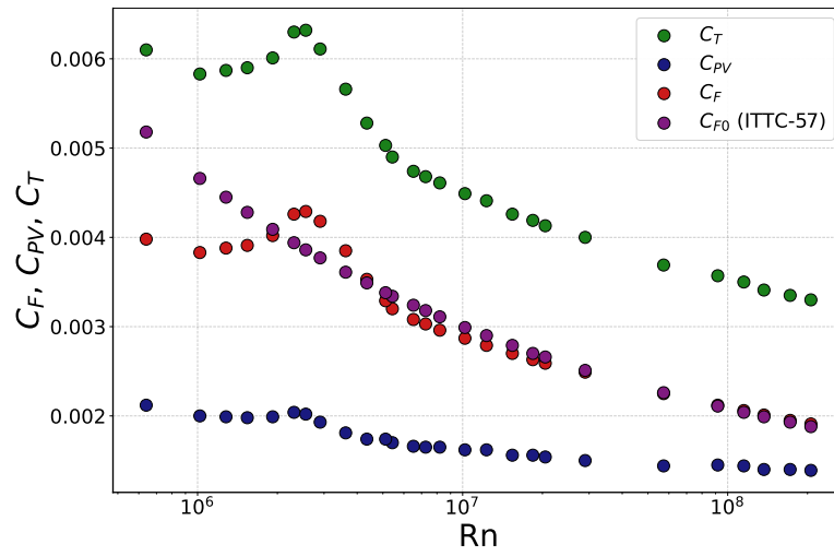
Figura 4.1.25: Coeficientes C_T , C_{PV} y C_F obtenidos mediante CFD en configuración de doble cuerpo, junto con la línea ITTC-57 ( C_{F0} ), en función de R_n para el P1 .
