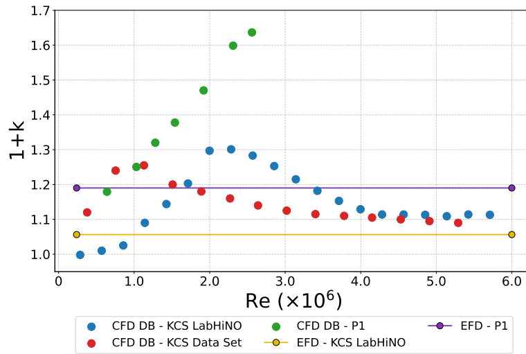
Figura 4.1.21: (1+k) frente a R_n para el KCS (CFD DB, escalas 1:79 y 1:75 de Terziev et al. [2021], y EFD a 1:79) y para el P1 (CFD DB y EFD, escala 1:20, Calado 3).
