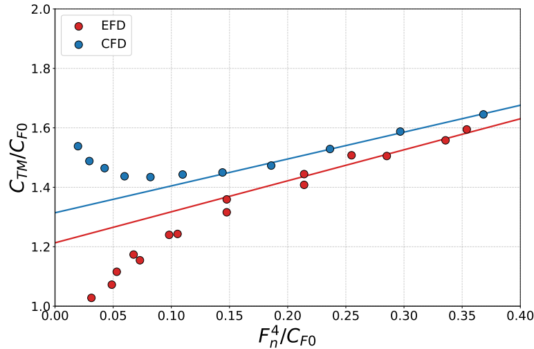
Figura 4.1.17: Diagrama de Prohaska del P1 comparando EFD y CFD. Calado 2.
