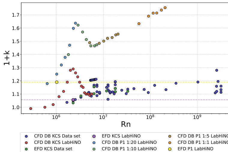
Figura 4.1.22: (1+k) frente a R_n para el KCS y el P1 , en escala logarítmica. Para el KCS se muestran los resultados propios obtenidos en el LabHiNO (CFD DB y Prohaska EFD, escala 1:79) junto con el conjunto de datos recopilado por Terziev et al. [2020] (CFD DB y Prohaska, otras escalas y laboratorios). Para el P1 se muestran únicamente resultados propios: CFD DB en las escalas 1:20, 1:10, 1:5 y 1:1, y el valor experimental obtenido por Prohaska en el LabHiNO (escala 1:20).
