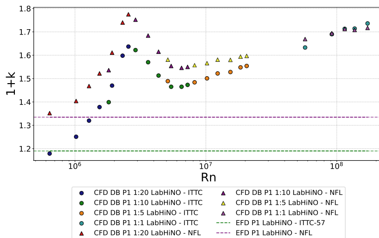
Figura 4.4.1: Variación de (1+k) en función de R_n para el P1 empleando la línea ITTC-57 y la NFL de Korkmaz et al. [2019].
