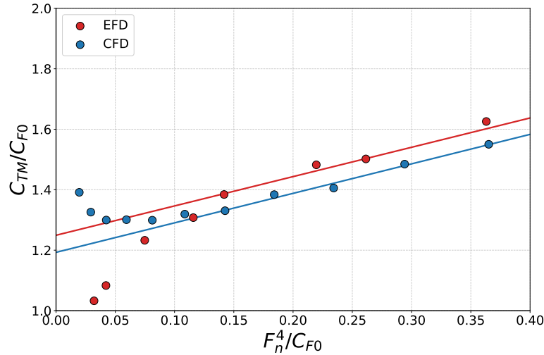
Figura 4.1.16: Diagrama de Prohaska del P1 comparando EFD y CFD. Calado 1.
