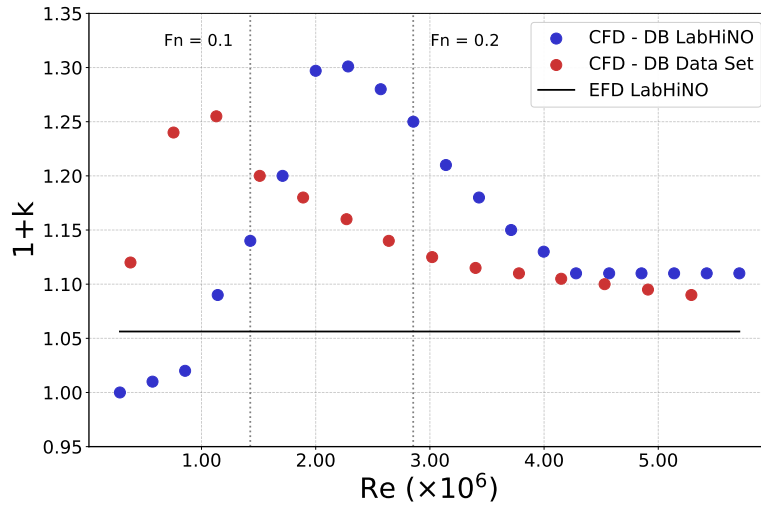
Figura 4.1.13: Comparación de 1 + k numérico vs R_n para el KCS 1:79 (escala LabHiNO) y 1:75 [Terziev et al., 2021].
