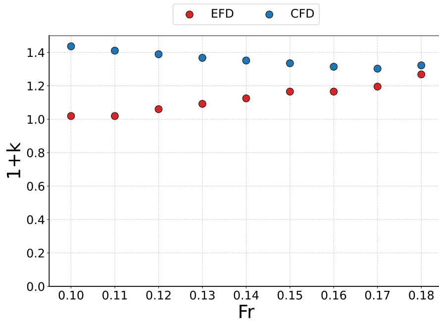
Figura 4.1.27: Variación del factor de forma ( 1+k ) del P1 para el Calado 0.180 m (T2), obtenido mediante el método de Prohaska a partir de EFD y CFD, en función del límite inferior del rango de Froude considerado en el ajuste.
