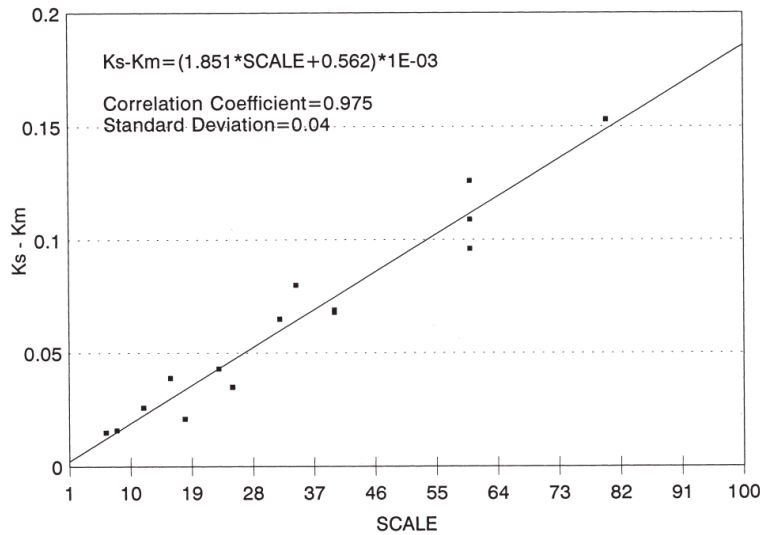
Figura 2.3.1: Efecto de escala del factor de forma en función de la razón de escala. Adaptado de García-Gómez [2000].
