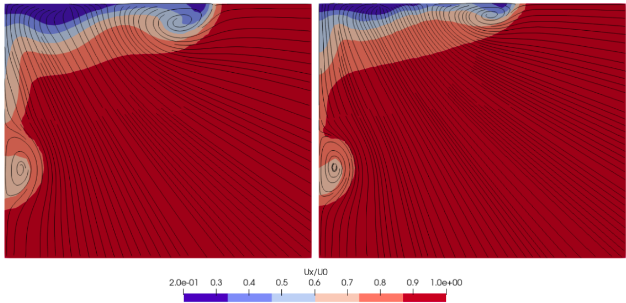
Figura 4.1.39: Contornos de velocidad longitudinal U_x/U_0 en un plano transversal ubicado a 0.05 L_{WL} aguas abajo del espejo, para escala modelo, 1:20 (izquierda, \log(Re) \approx 6 ) y escala buque, 1:1 (derecha, \log(Re) \approx 8 ), a Fr = 0.2 y calado 0.195 m (T3). En cada panel, el borde izquierdo corresponde al plano de crujía y la parte superior se ubica hacia la superficie libre. Foco inferior: vórtice de quilla; foco superior: vórtice de pantoque.
