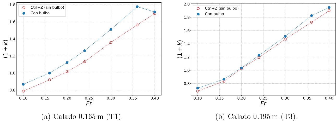
Figura 4.2.4: Factor de forma (1 + k) del P1 con y sin proa bulbo, obtenido mediante el método de doble cuerpo (DB), en función del número de Froude, para ambos calados.
