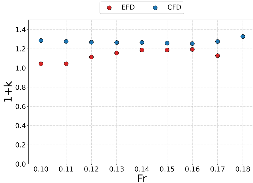
Figura 4.1.28: Variación del factor de forma ( 1+k ) del P1 para el Calado 0.195 m (T3), obtenido mediante el método de Prohaska a partir de EFD y CFD, en función del límite inferior del rango de Froude considerado en el ajuste.
