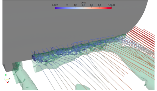
(d) Escala buque, Fr = 0.36
