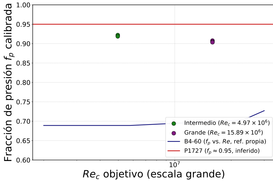
Figura 5.4.5: Fracción de presión calibrada en los dos puntos de escala independientes, comparada con la curva propia de la B4-60 (evaluada en función de Re ) y con el valor inferido del P1727.
