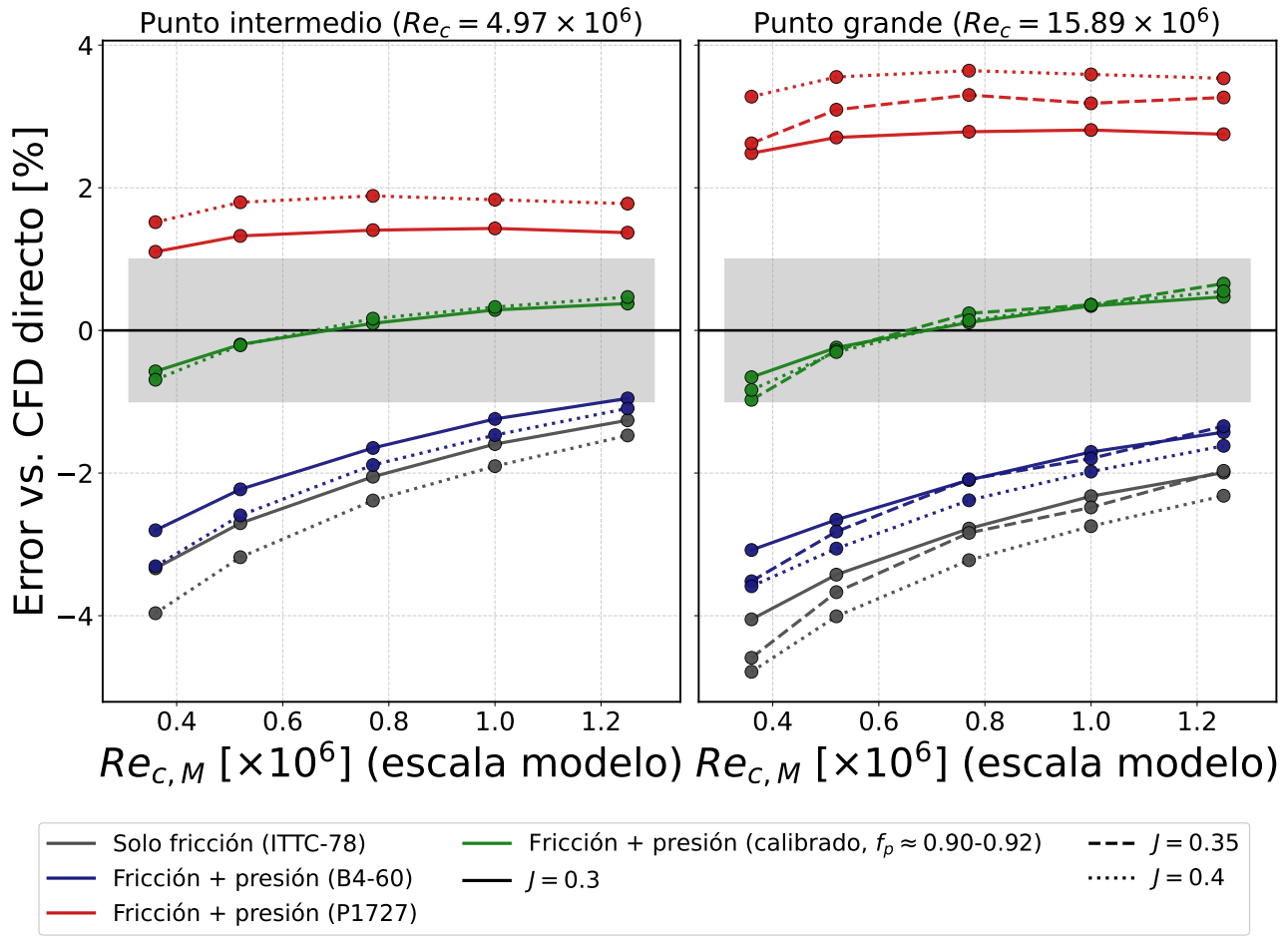
Figura 5.4.6: Error de la extrapolación Fully Turbulent respecto de los dos puntos de validación, para las tres correcciones evaluadas y los tres J calculados.
