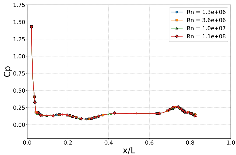
Figura 4.1.46: Distribución de C_P(x/L) sobre el plano |z|/T = 0.5 .
