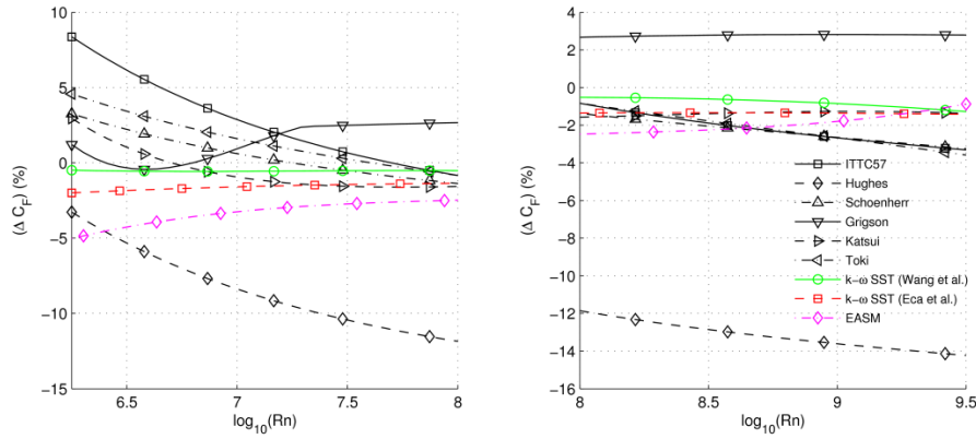
Figura 2.1.1: Comparación del coeficiente de fricción C_F en función del número de Reynolds para distintas líneas de fricción numéricas (NFL k - \omega SST de Wang et al. [2015], NFL k - \omega SST de Eça and Hoekstra [2008] y NFL EASM de Korkmaz et al. [2019]) tomando la línea ITTC-57 como referencia. Adaptado de Korkmaz [2023].
