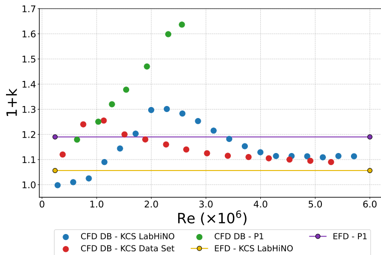
Figura 4.1.21: (1+k) frente a Re para el KCS (CFD DB, escalas 1:79 y 1:75 de Terziev et al. [2021], y EFD a 1:79) y para el P1 (CFD DB y EFD, escala 1:20, Calado 3).
