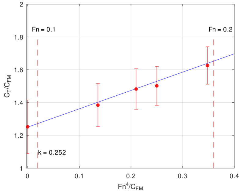
Figura 4.1.4: Ajuste lineal con ponderación mediante el método de York aplicado al P1 para la estimación de (1+k) y su incertidumbre. Calado 1.
