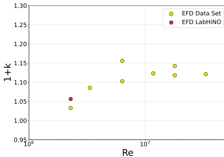
Figura 4.1.7: Comparación del factor de forma (1 + k) del KCS obtenido en el LabHiNO (punto rojo) con resultados experimentales históricos del KCS compilados de literatura internacional por Terziev et al. [2020] (puntos amarillos), en función del número de Reynolds.
