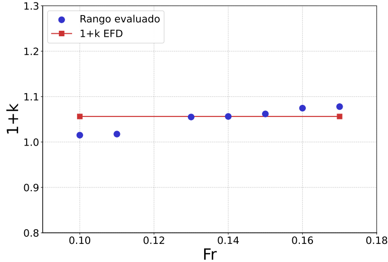
Figura 4.1.6: Variación del factor de forma (1 + k) para el modelo KCS en función del límite inferior del rango de Froude utilizado en el ajuste de Prohaska, con límite superior fijo en Fr = 0,20 . El cuadrado rojo indica el valor adoptado.
