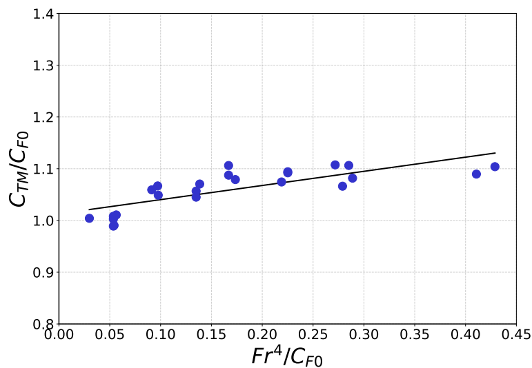
Figura 4.1.5: Diagrama de Prohaska para el modelo KCS. Se grafica C_{TM}/C_{F0} frente a Fr^4/C_{F0} , donde C_{F0} es el coeficiente de fricción de placa plana al Re del modelo según la línea ITTC-57. La línea continua representa el ajuste por mínimos cuadrados, cuya extrapolación al origen permite obtener el valor de 1 + k .
