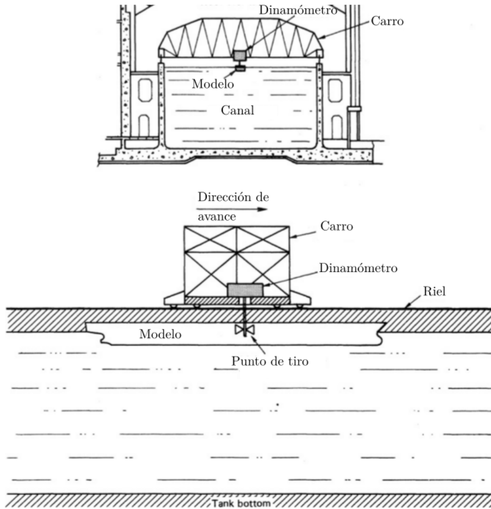
Figura 3.2.5: Esquema del montaje del ensayo de resistencia. Adaptado de Molland [2011].
