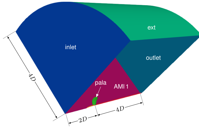
Figura 3.4.3: Dominio computacional empleado en las simulaciones (sector de 90° con interfaz periódica AMI). Las distancias se expresan en diámetros de hélice D .
