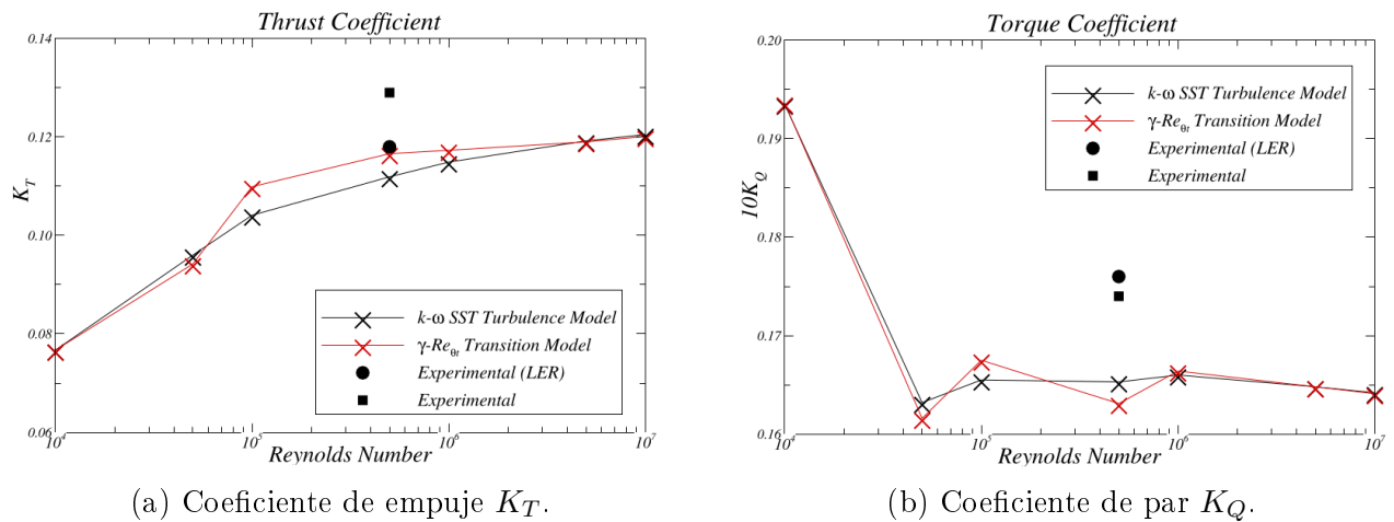
Figura 2.4.1: Variación no monótona de los coeficientes de empuje y de par con el número de Reynolds seccional Re_{c,0,7R} , mostrando la joroba característica del régimen transicional [Baltazar et al., 2018].
