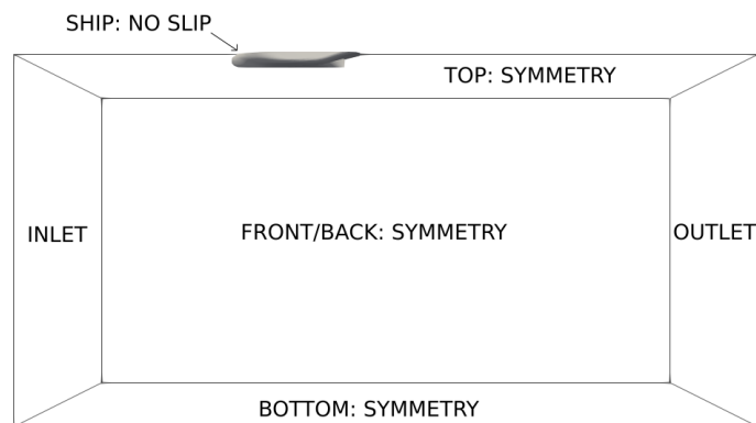
Figura 4.1.18: Dominio reducido para simulación sin superficie libre.
