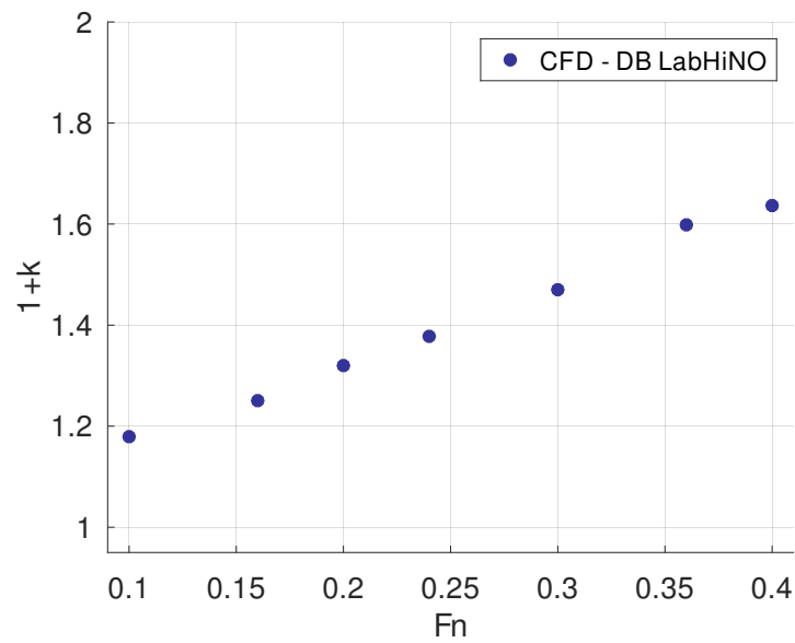
Figura 4.1.21: Factor de forma por método de doble cuerpo para el pesquero. Calado 3.
