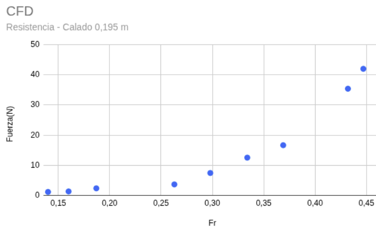
Figura 4.1.15: Resistencia al avance en función de Fr. Calado 3.
