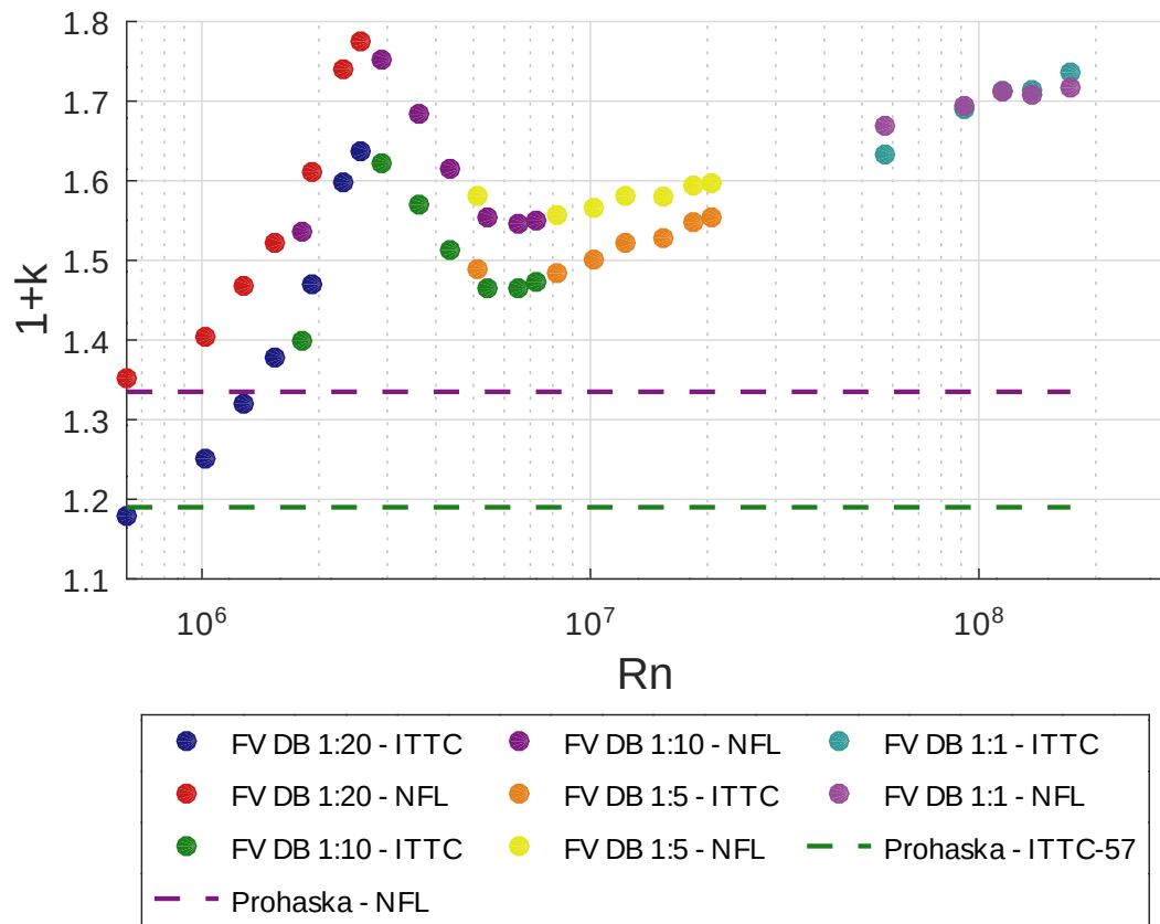
Figura 4.2.14: Variación de 1+k en función de Rn para el pesquero (FV) empleando dos líneas de fricción distintas.
