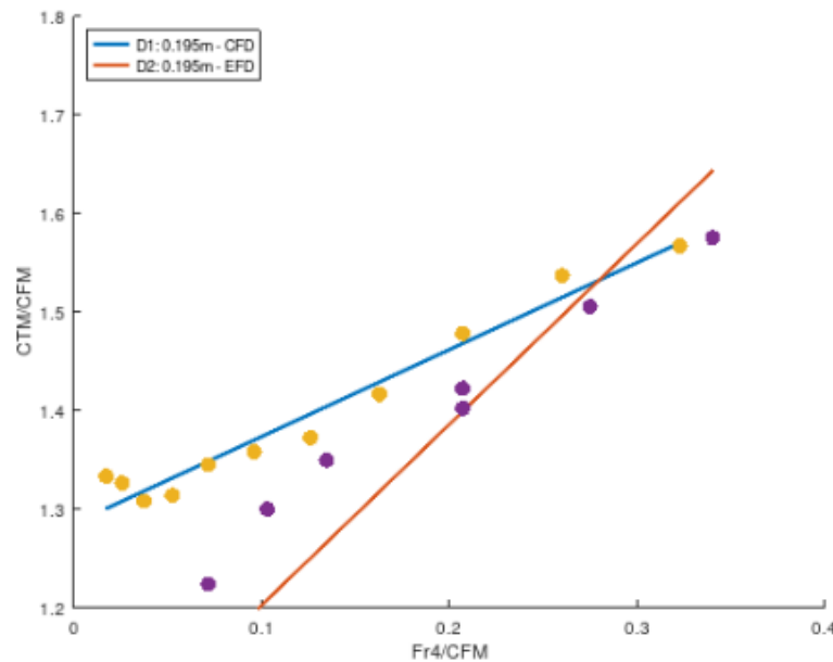
Figura 4.1.28: Resistencia al avance en función de Fr . Calado 2.
