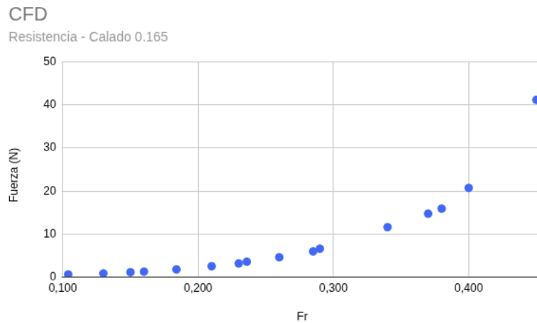
Figura 4.1.13: Resistencia al avance en función de Fr. Calado 1.
