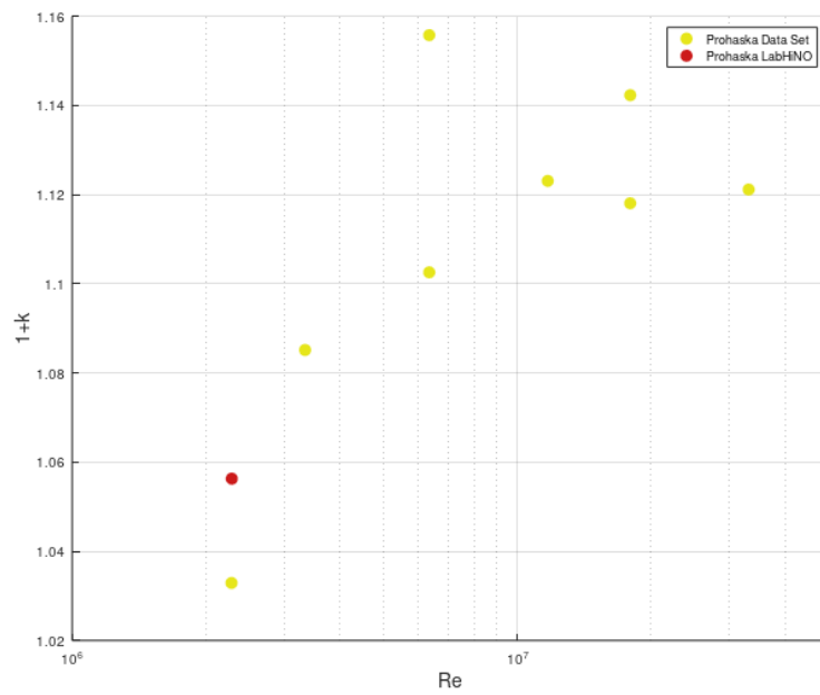
Figura 4.1.11: Comparación del factor de forma (1+k) del KCS obtenido en el LabHiNO con resultados internacionales.
