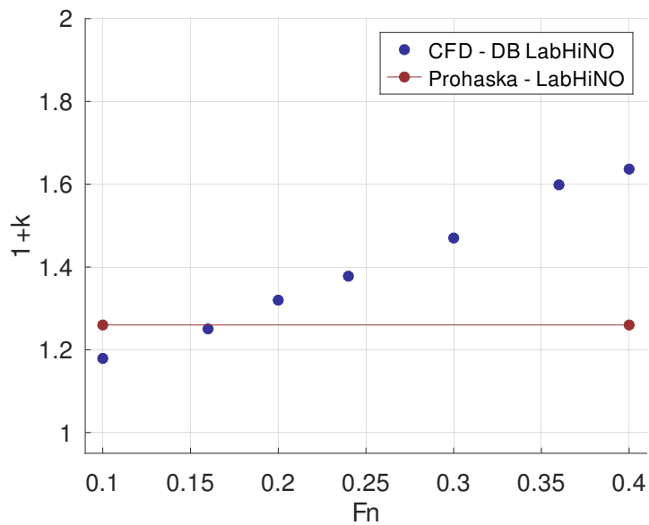
Figura 4.1.35: Comparación de factor de forma experimental y computacional adoptado con valores obtenidos por método de doble cuerpo. Calado 3.
