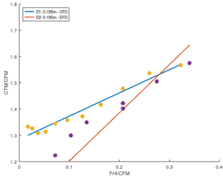
Figura 4.1.29: Resistencia al avance en función de Fr. Calado 3.
