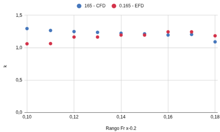
Figura 4.1.30: Variación del factor de forma experimental ( 1 + k ) para el pesquero TPA en función del rango de Froude utilizado en el ajuste de Prohaska. Calado 1.
