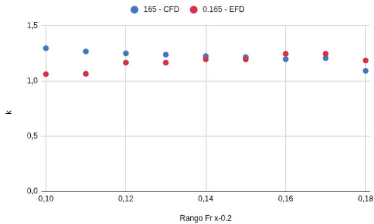
Figura 4.1.31: Variación del factor de forma experimental ( 1 + k ) para el pesquero TPA en función del rango de Froude utilizado en el ajuste de Prohaska. Calado 2.
