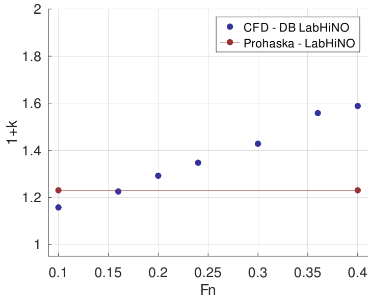
Figura 4.1.34: Comparación de factor de forma experimental y computacional adoptado con valores obtenidos por método de doble cuerpo. Calado 2.
