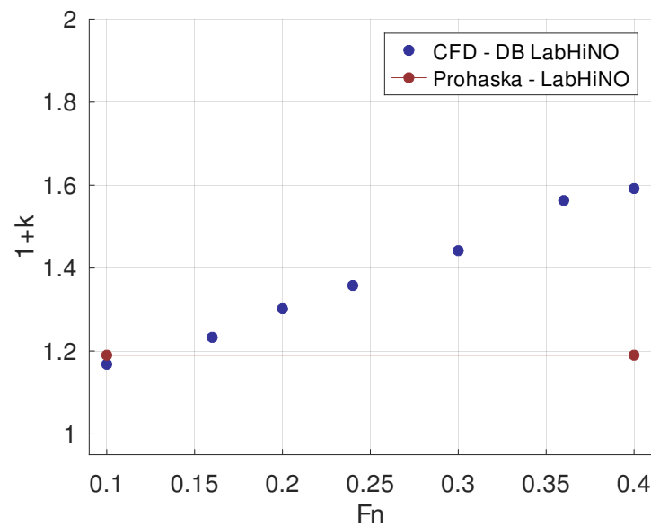
Figura 4.1.33: Comparación de factor de forma experimental y computacional adoptado con valores obtenidos por método de doble cuerpo. Calado 1.
