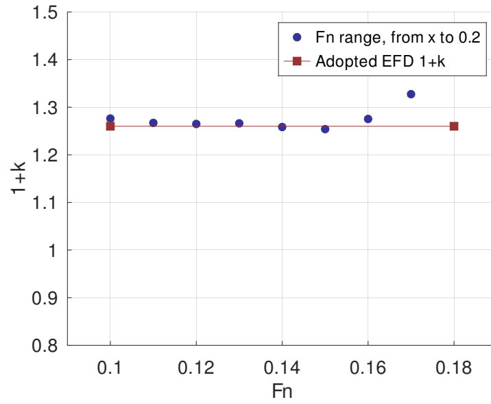
Figura 4.1.17: Variación del factor de forma experimental ( 1 + k ) para el pesquero TPA en función del rango de Froude utilizado en el ajuste de Prohaska. Calado 0.195
