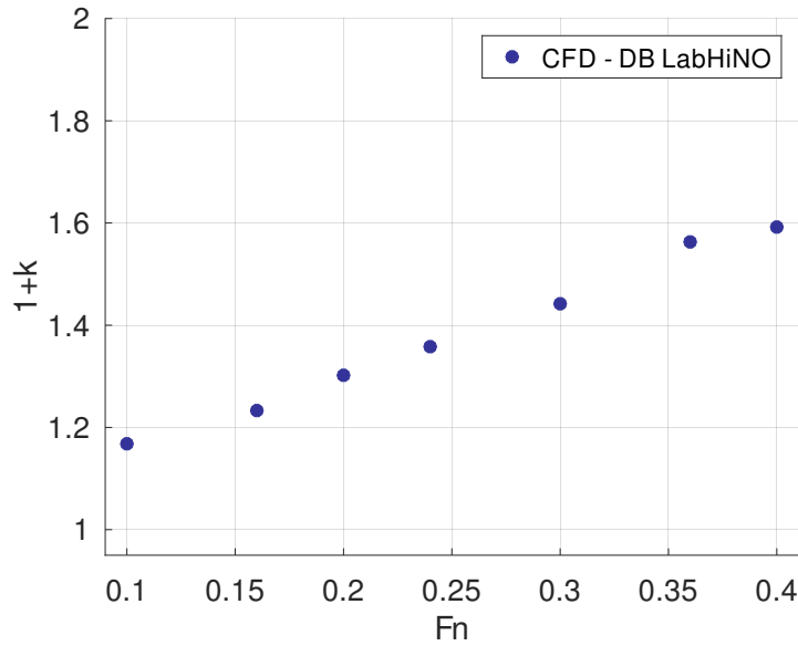
Figura 4.1.19: Factor de forma por método de doble cuerpo para el pesquero. Calado 1.
