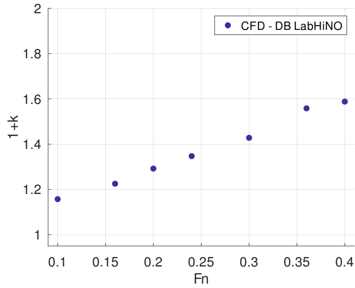
Figura 4.1.20: Factor de forma por método de doble cuerpo para el pesquero. Calado 2.
