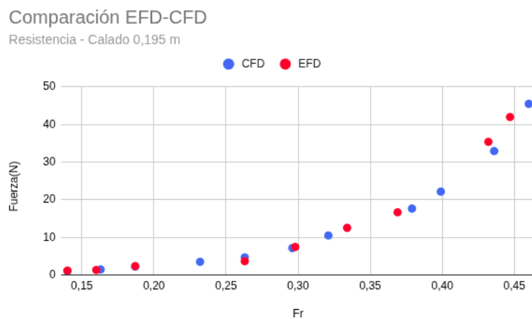
Figura 4.1.26: Resistencia al avance en función de Fr. Calado 1.
