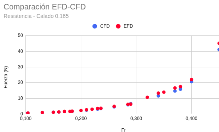
Figura 4.1.24: Resistencia al avance en función de Fr . Calado 1.
