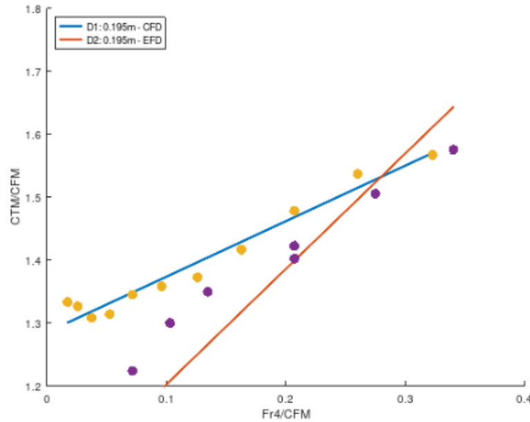
Figura 4.1.27: Resistencia al avance en función de Fr . Calado 1.
