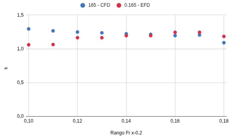
Figura 4.1.32: Variación del factor de forma experimental ( 1 + k ) para el pesquero TPA en función del rango de Froude utilizado en el ajuste de Prohaska. Calado 3.
