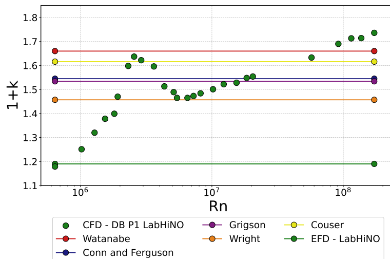
Figura 4.6.1: Valores de (1 + k) para el P1 en función de R_n , obtenidos por CFD DB, EFD y correlaciones empíricas de la literatura [Molland et al., 2017, Conn and Ferguson, 1968, Grigson, 2000, Wright, 1984, Couser et al., 1997].
