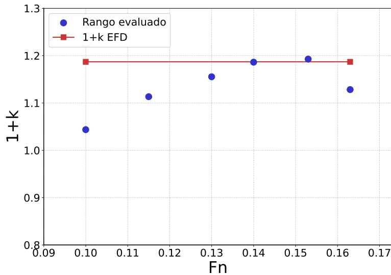
Figura 4.1.3: Variación del factor de forma (1+k) al modificar el límite inferior del rango de Froude (puntos azules), manteniendo el superior en F_n = 0,20 . La línea roja indica el valor de (1+k) adoptado mediante el método de Prohaska en el rango 0,15 < F_n < 0,20 . Calado 3; comportamiento análogo en otros calados.
