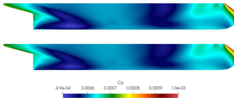
Figura 4.1.43: C_P para Fr = 0,2 , vista lateral. Arriba: escala 1:20. Abajo: escala 1:1.
