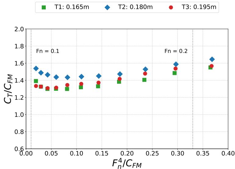
Figura 4.1.10: Diagramas del método de Prohaska para los tres calados del P1 . La desviación respecto de la linealidad teórica se acentúa a bajas números de Froude.
