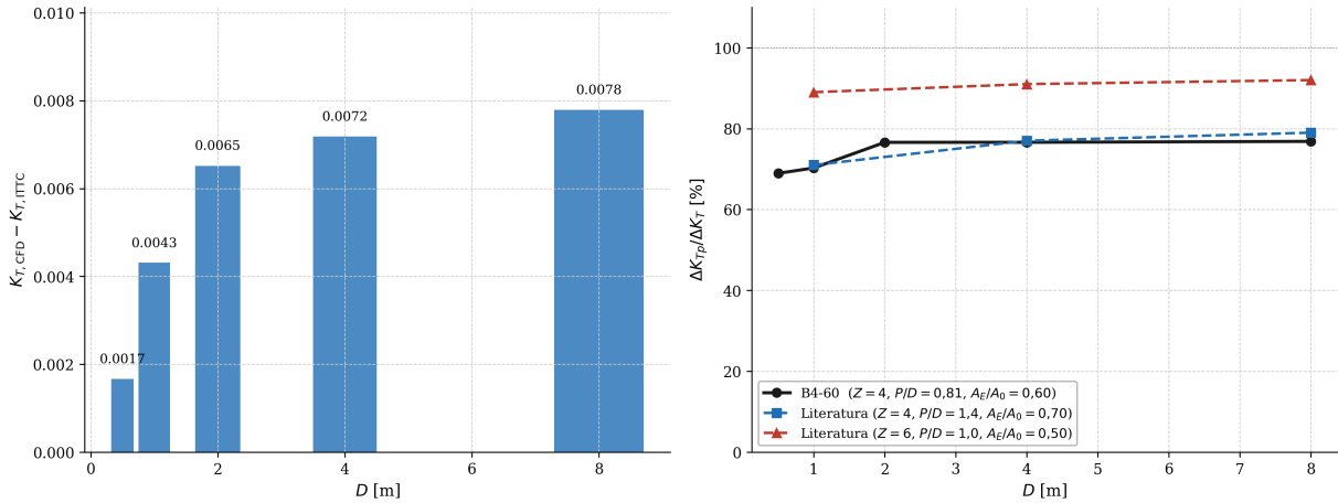
Figura 5.3.7: Izquierda: diferencia K_{T,CFD} - K_{T,ITTC} en función del diámetro. Derecha: fracción del efecto de escala en K_T atribuible a la componente de presión ( \Delta K_{Tp}/\Delta K_T ), comparada con datos de la literatura para otras geometrías.
