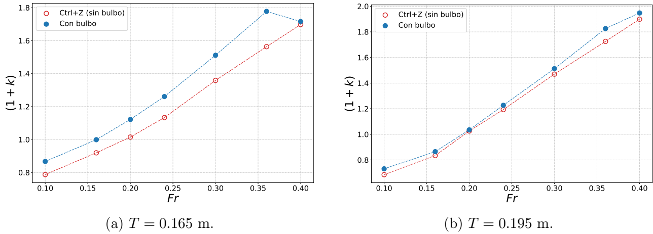
Figura 4.2.6: Factor de forma (1+k) del P1 con y sin proa bulbo en función del número de Froude, para ambos calados.
