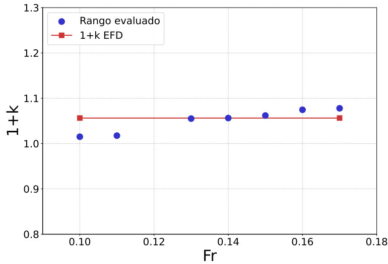
Figura 4.1.7: Variación del factor de forma ( 1 + k ) para el modelo KCS en función del límite inferior del rango de Froude utilizado en el ajuste de Prohaska, con límite superior fijo en Fr = 0,20 . El cuadrado rojo indica el valor adoptado.
