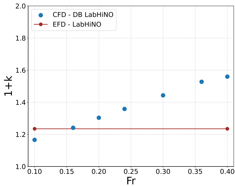
Figura 4.1.29: Comparación entre el valor de (1 + k) adoptado por Prohaska (línea horizontal roja) y los valores obtenidos mediante el método de doble cuerpo (DB) en función de Fr (puntos azules) para el P1 , Calado 1.
