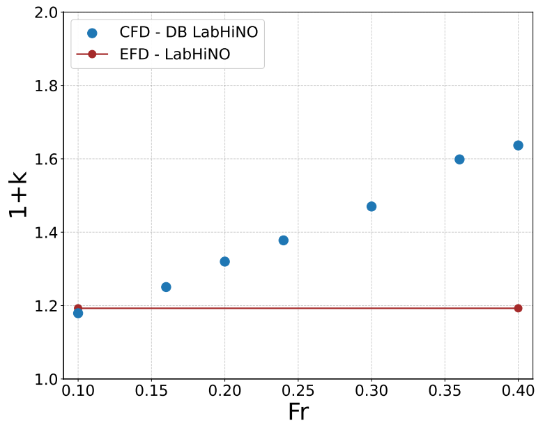
Figura 4.1.31: Comparación entre el valor de (1 + k) adoptado por Prohaska (línea horizontal roja) y los valores obtenidos mediante el método de doble cuerpo (DB) en función de Fr (puntos azules) para el P1 , Calado 3.
