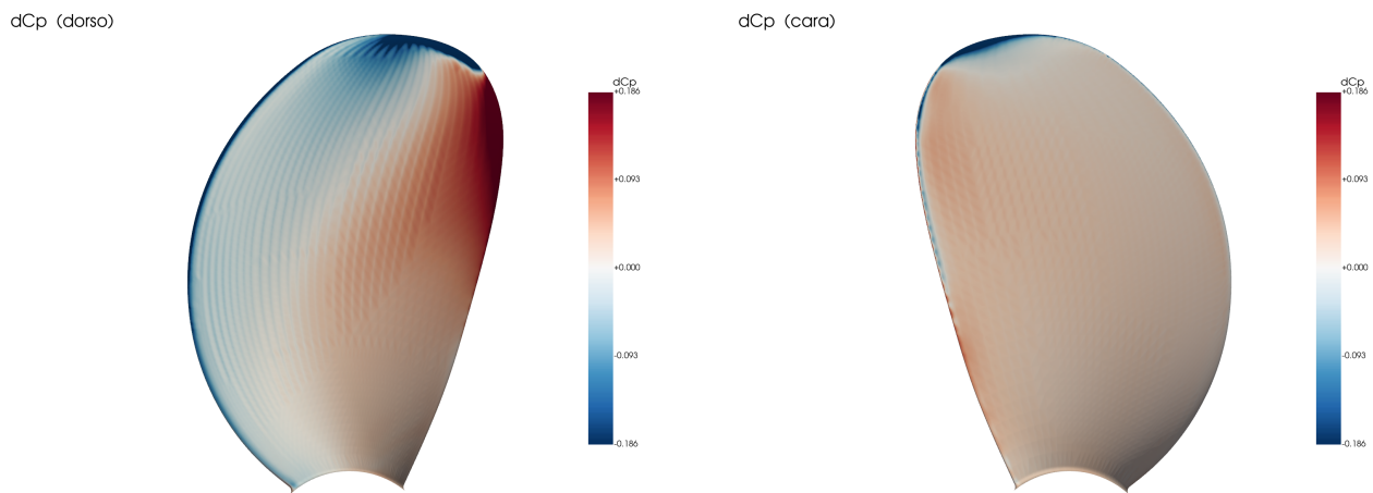
Figura 5.3.3: Campo de diferencia \Delta C_p = C_p(Re_n) - C_p(Re_{n,\text{ref}}) entre la escala modelo y Re_n \approx 2,5 \times 10^6 , sobre el dorso (izquierda, lado de succión) y la cara (derecha, lado de presión) de la pala B4-60. El rango de color es simétrico y se recorta al percentil 98 de |\Delta C_p| para evitar que los extremos de punta y bordes dominen la escala.
