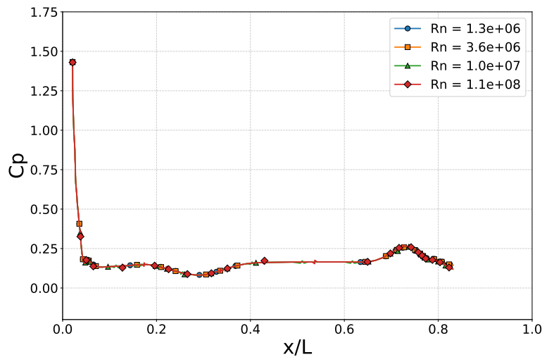
Figura 4.1.45: Distribución de C_P(x/L) sobre el plano z/T = 0.5 .
