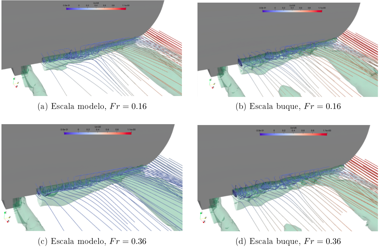
Figura 4.3.3: Comparación de la recirculación en popa sumergida para distintas escalas y números de Froude (calado 0.195 m). Casos sin superficie libre.
