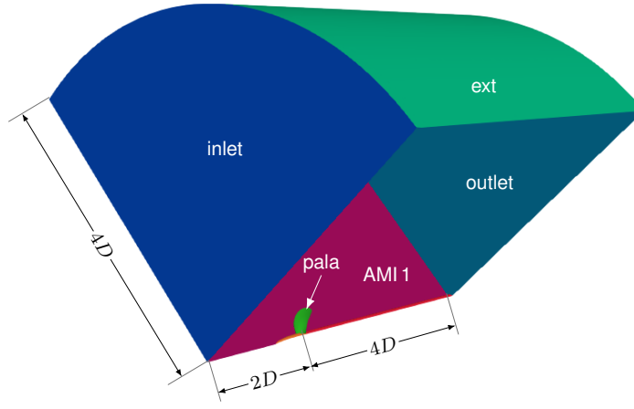
Figura 3.5.1: Dominio computacional empleado en las simulaciones (sector de 90° con interfaz periódica AMI). Las distancias se expresan en diámetros de hélice D .
