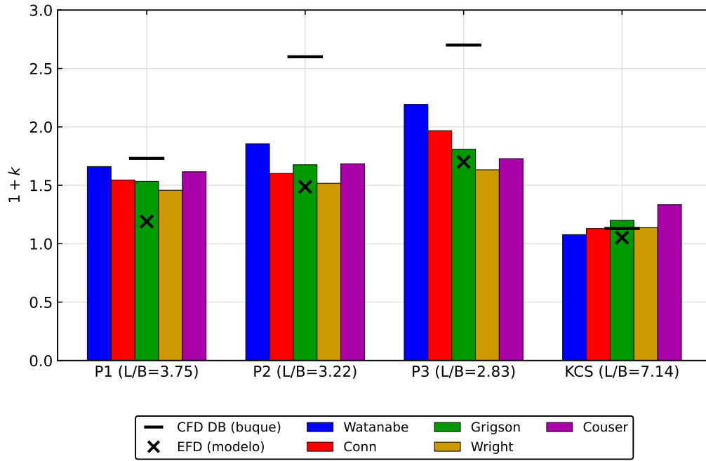
Figura 4.6.2: Correlaciones empíricas de (1+k) aplicadas al P1 , el P2 , el P3 y el KCS , comparadas con el valor CFD DB a escala buque (guion horizontal) y el valor EFD a escala modelo (cruz) de cada casco.
