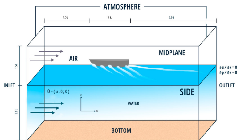
Figura 3.4.1: Dominio computacional y condiciones de contorno para las simulaciones de resistencia con superficie libre.
