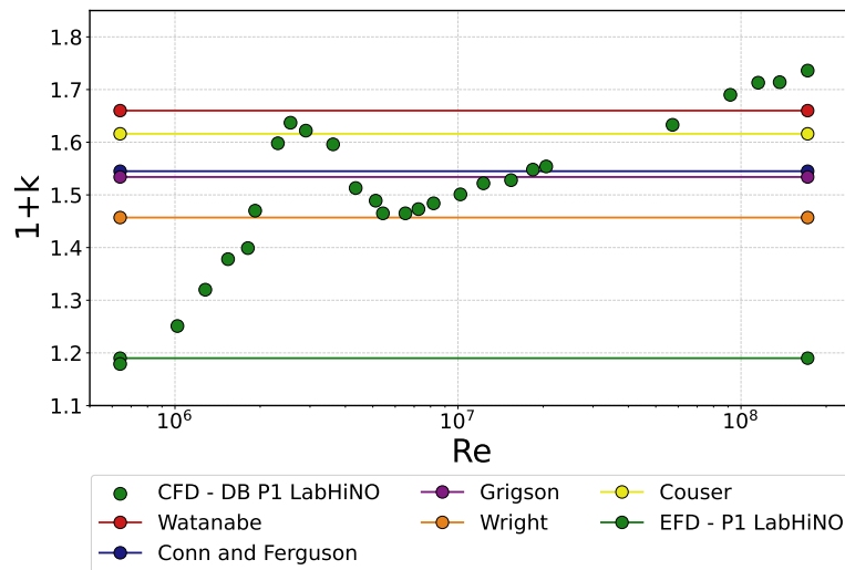
Figura 4.6.1: Valores de (1+k) para el P1 en función de Re , obtenidos por CFD DB, EFD y correlaciones empíricas de la literatura [Molland et al., 2017, Conn and Ferguson, 1968, Grigson, 2000, Wright, 1984, Couser et al., 1997].
