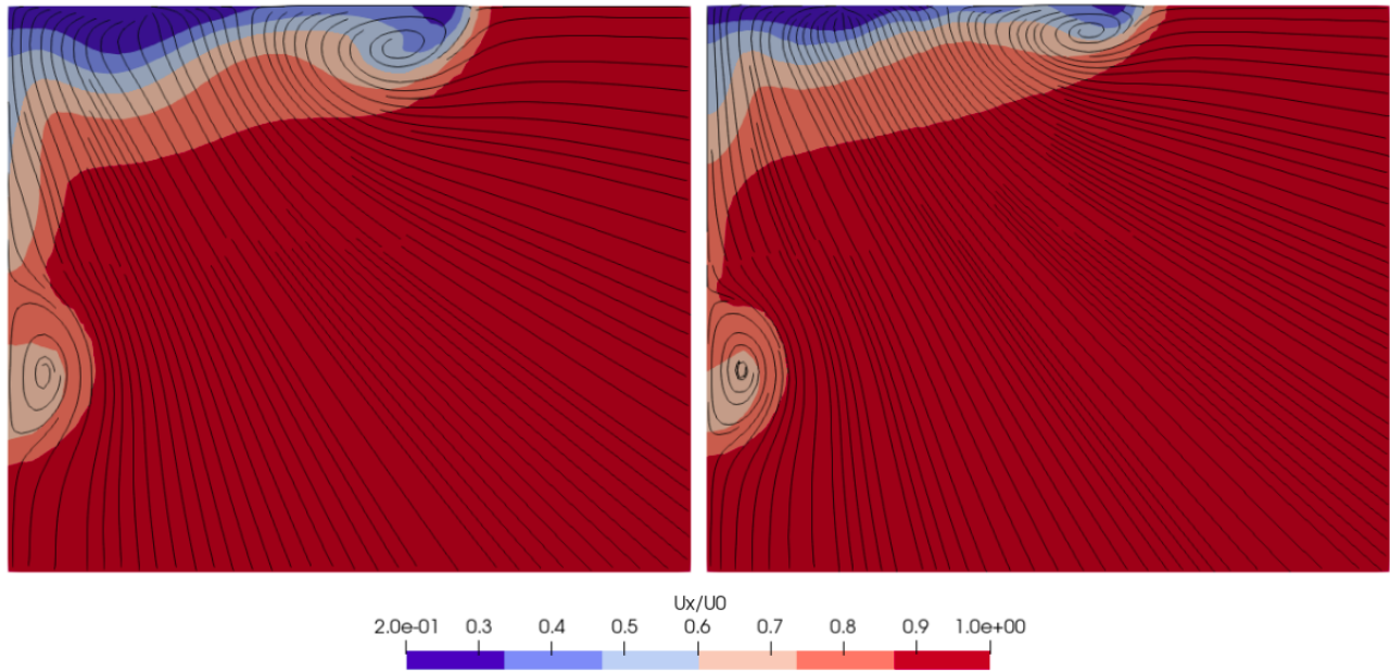
Figura 4.1.38: Contornos de velocidad longitudinal U_x/U_0 en un plano ubicado en x/L = 0.05 para escala modelo, 1:20 (izquierda, \log(Re) \approx 6 ) y escala buque, 1:1 (derecha, \log(Re) \approx 8 ), a Fr = 0.2 .
