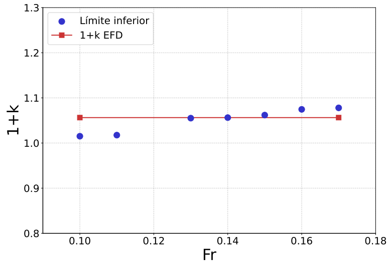
Figura 4.1.9: Variación del factor de forma (1+k) para el modelo KCS en función del límite inferior del rango de Froude utilizado en el ajuste de Prohaska, con límite superior fijo en Fr = 0.20 . El cuadrado rojo indica el valor adoptado.
