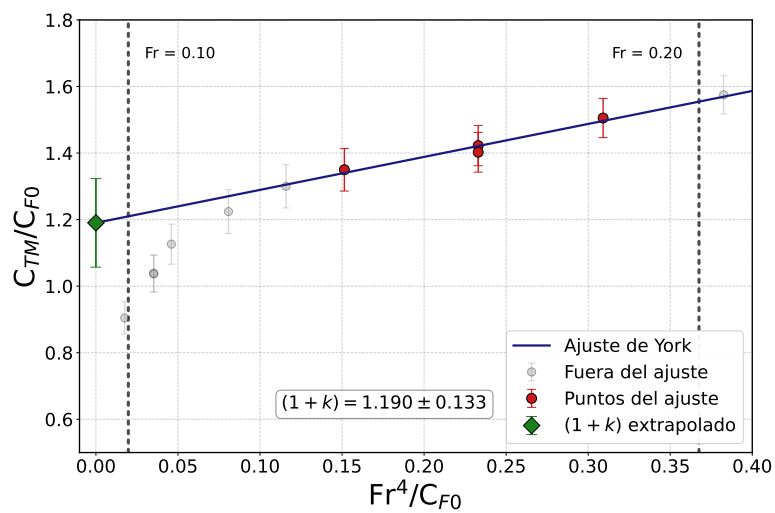
Figura 4.1.6: Ajuste lineal con ponderación mediante el método de York aplicado al P1 para la estimación de (1+k) y su incertidumbre. Las líneas verticales punteadas indican Fr = 0.10 y Fr = 0.20 para el P1 .
