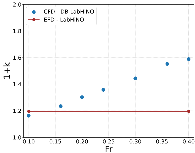
Figura 4.1.30: Comparación entre el valor de (1 + k) adoptado por Prohaska (línea horizontal roja) y los valores obtenidos mediante el método de doble cuerpo (DB) en función de Fr (puntos azules) para el P1 , Calado 2.
