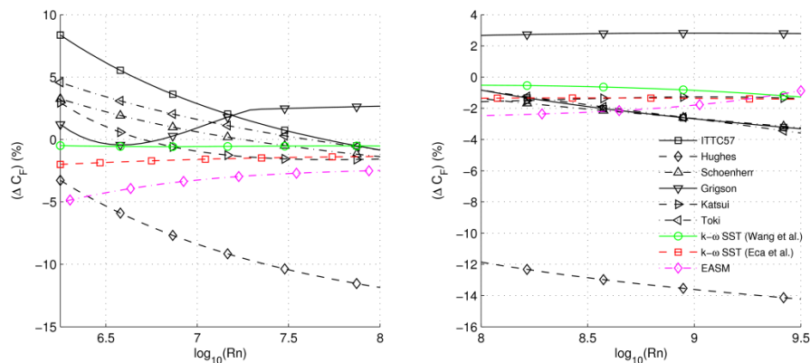
Figura 2.2.1: Líneas de fricción numéricas frente a la línea ITTC-57. Adaptado de Korkmaz [2023].
