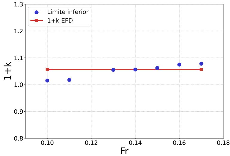
Figura 4.1.9: Variación del factor de forma ( 1+k ) para el modelo KCS en función del límite inferior del rango de Froude utilizado en el ajuste de Prohaska, con límite superior fijo en Fr = 0.20 . El cuadrado rojo indica el valor adoptado.
