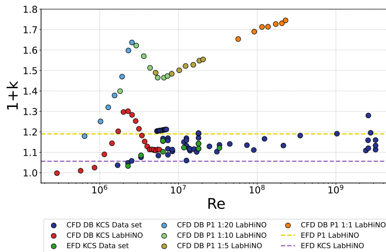
Figura 4.1.33: (1+k) frente a Re para el KCS y el P1 , en escala logarítmica. Para el KCS se muestran los resultados propios obtenidos en el LabHiNO (CFD DB y Prohaska EFD, escala 1:79) junto con el conjunto de datos recopilado en Terziev et al. [2020] (CFD DB y Prohaska, otras escalas y laboratorios). Para el P1 se muestran únicamente resultados propios: CFD DB en las escalas 1:20, 1:10, 1:5 y 1:1, y el valor experimental obtenido por Prohaska en el LabHiNO (escala 1:20).
