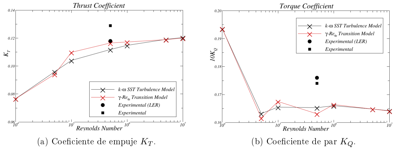
Figura 2.5.1: Coeficientes de empuje y de par frente al número de Reynolds seccional Re_{c,0,7R} . Adaptado de Baltazar et al. [2018].
