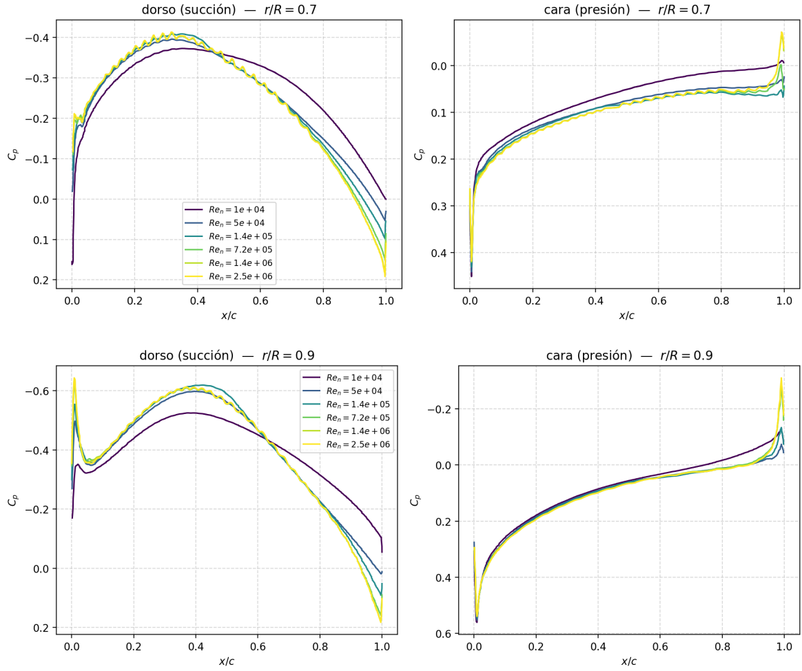
Figura 5.3.6: Distribución de C_p a lo largo de la cuerda ( x/c ) en las secciones r/R = 0,7 (arriba) y r/R = 0,9 (abajo), para las escalas del barrido, separada en dorso (succión, izquierda) y cara (presión, derecha). El eje de C_p está invertido (succión hacia arriba). Se aprecia el pico de succión de borde de ataque profundizándose con Re_n sobre el dorso y la escasa sensibilidad de la cara.
