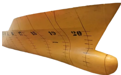
(a) Vista en perspectiva de proa. Se observan las marcas de calado y los estimuladores de turbulencia.
