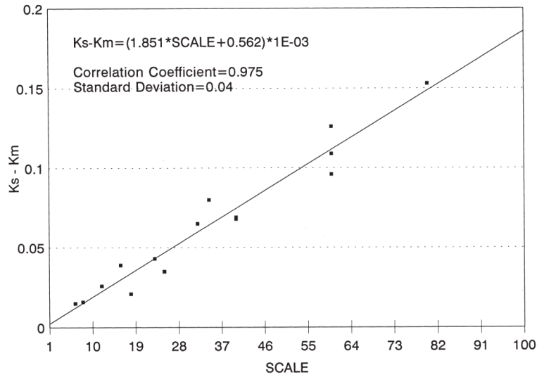
Figura 2.3.1: Efecto de escala del factor de forma en función de la razón de escala. Adaptado de Garcia-Gómez [2000].
