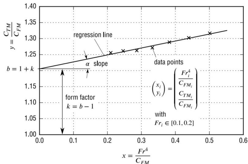
Figura 2.1.1: Diagrama del método de Prohaska. Adaptado de Birk [2019].
