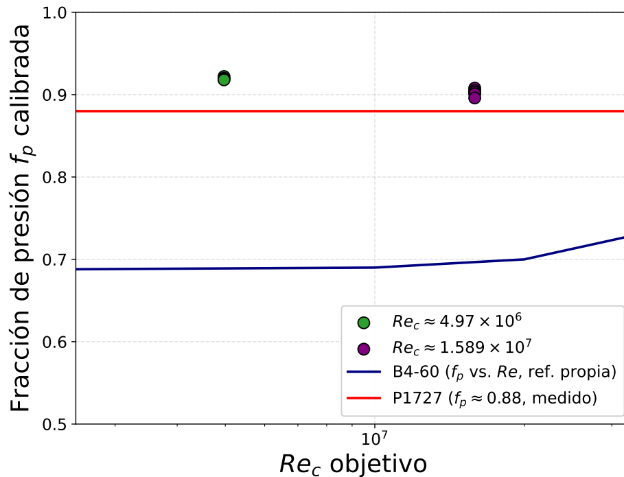
Figura 5.4.6: Fracción de presión calibrada en los dos puntos de escala independientes, comparada con la curva propia de la B4-60 (evaluada en función de Re ) y con el valor inferido del P1727.
