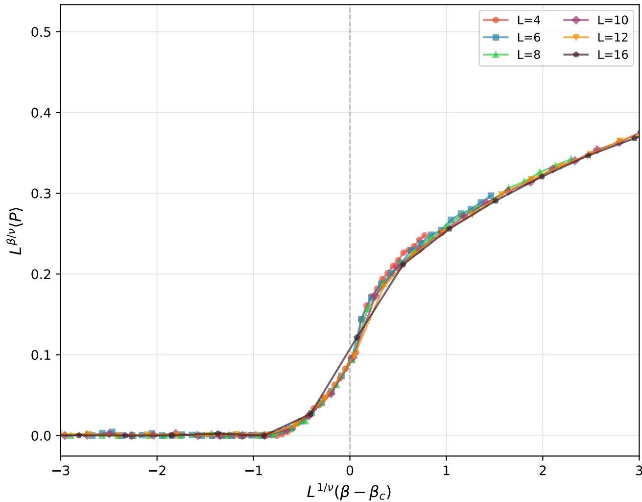
(b) Order Parameter Collapse \beta=0.327
