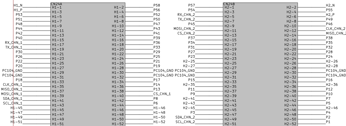
PC104 slot N°4
