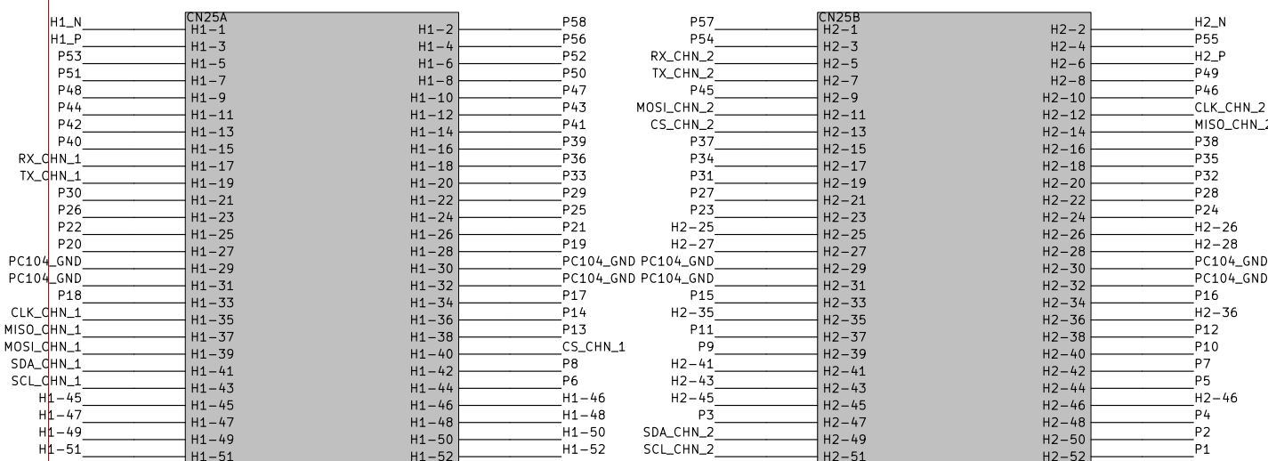
PC104 slot N°1
