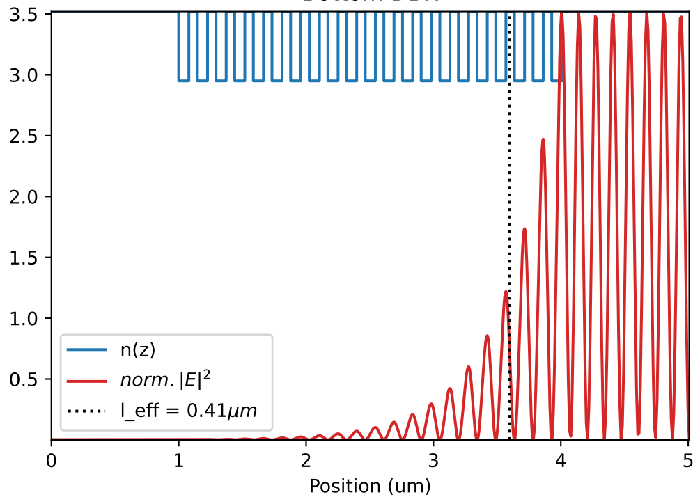
Bottom DBR
