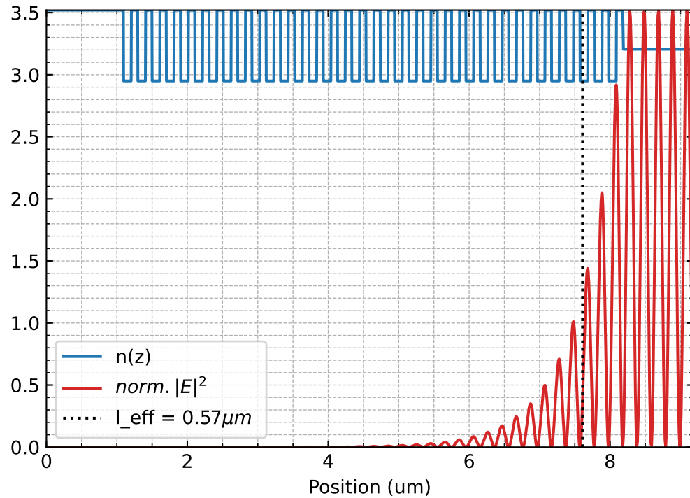
Bottom DBR
