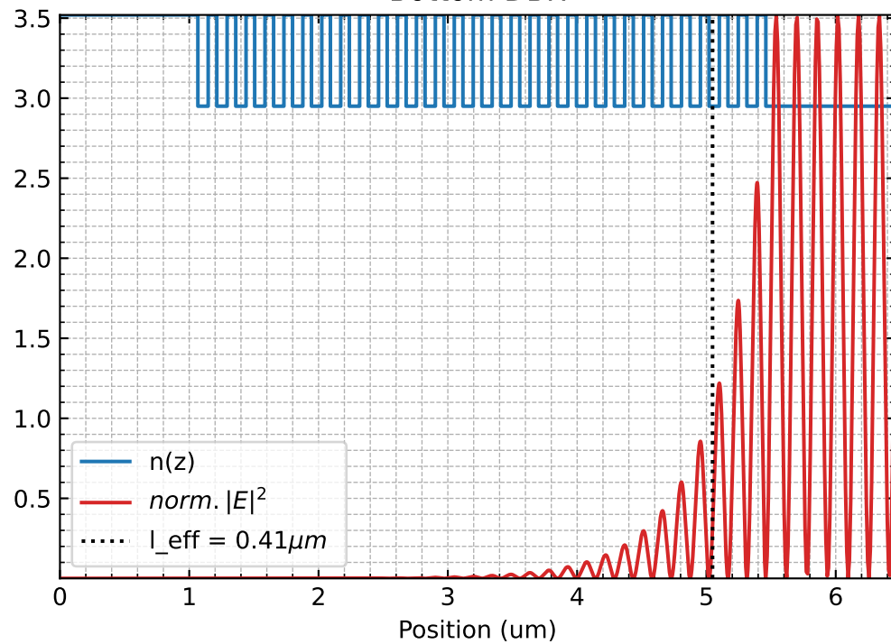
Bottom DBR
