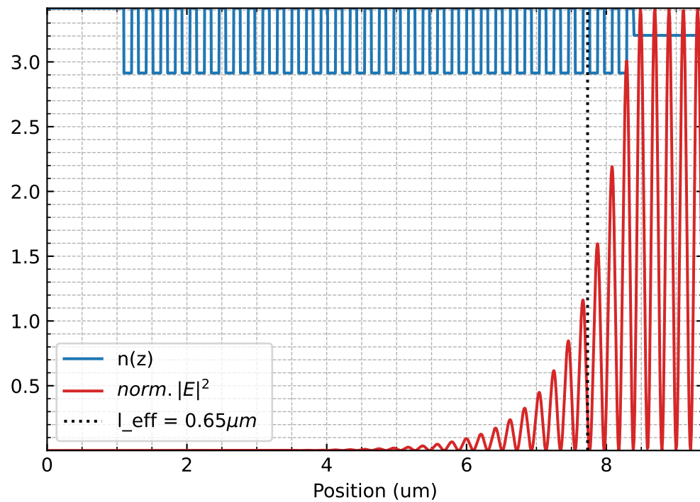
Bottom DBR
