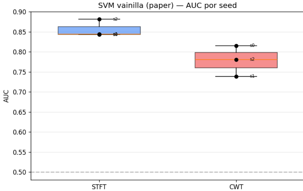
Figura 1: Distribución de AUC por sujeto-test (LOSO) para SVM vainilla, agregada a través de 3 seeds.
