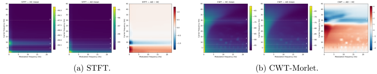
Figura 4: Espectrogramas de modulación promedio (AD vs HC) bajo STFT y CWT. La presentación 45 \times 45 oculta el desajuste en el rango del eje de modulación (Nyquist 1,56 Hz vs 100 Hz).
