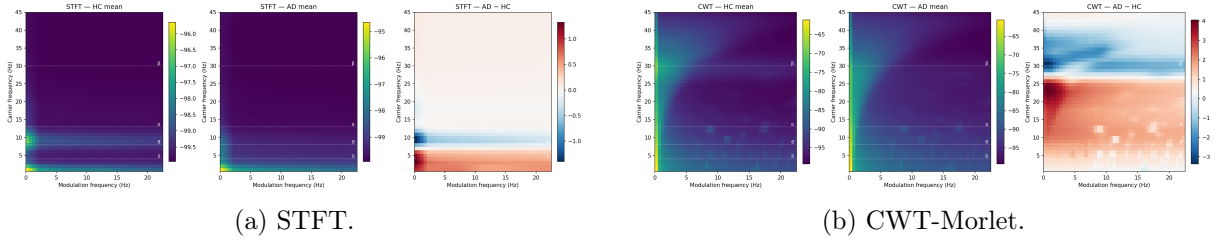
Figura 6: Espectrogramas de modulación promedio (AD vs HC) bajo STFT y CWT. La presentación 45 \times 45 oculta el desajuste en el rango del eje de modulación (Nyquist 1,56 Hz vs 100 Hz).
