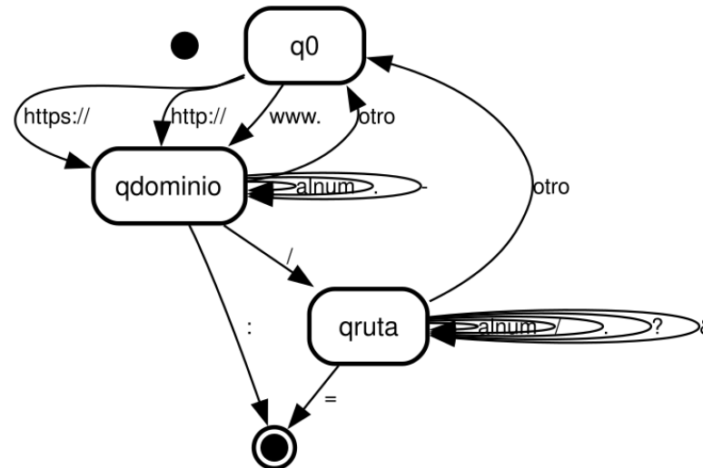
Figura 3: Diagrama de estados del UrlAutomaton.
