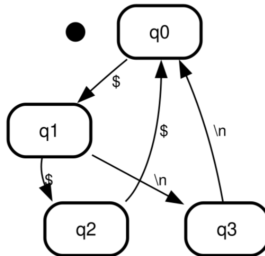
Figura 1: Diagrama de estados del CommandAutomaton.
