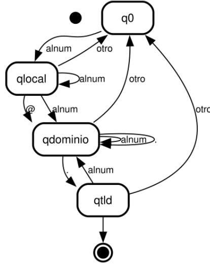
Figura 2: Diagrama de estados del EmailAutomaton.
