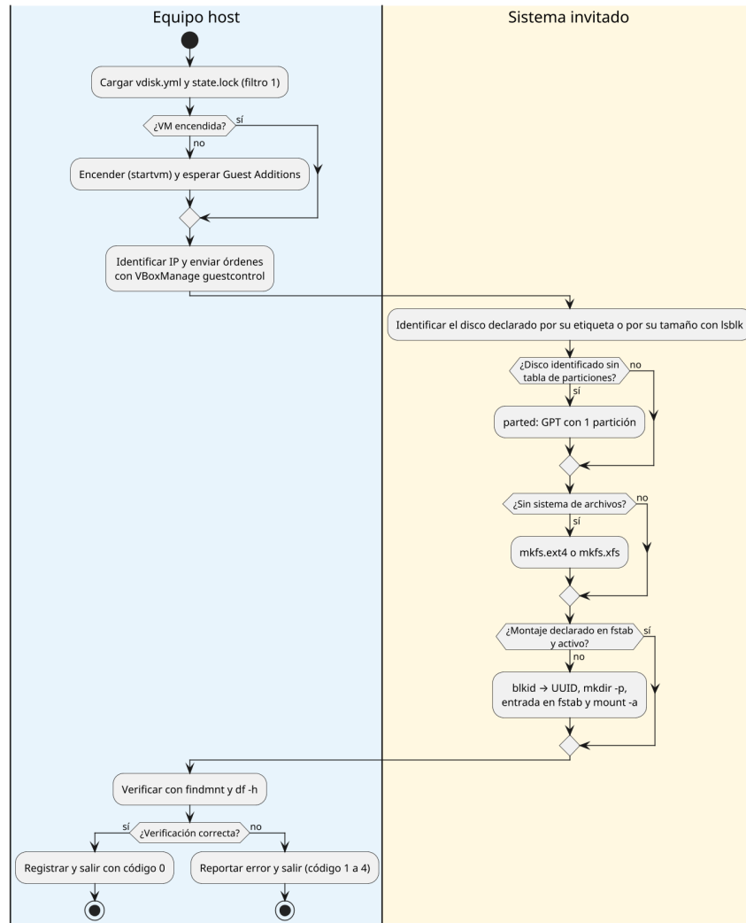
Figura 2: Diagrama de procesos de la automatización idempotente, con las etapas ejecutadas en el host y en el sistema invitado
