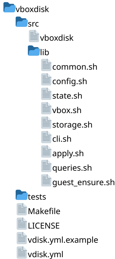
Figura 3: Árbol de ficheros de la solución, con el punto de entrada, las bibliotecas de src/lib/ y las pruebas de tests/
