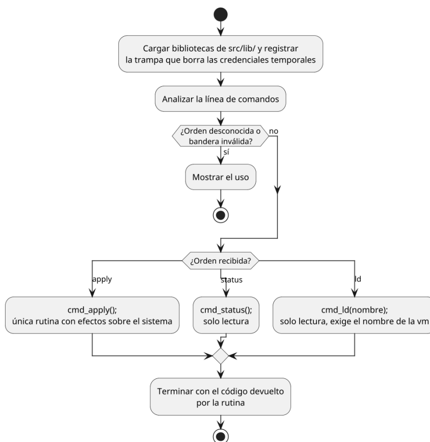
Figura 4: Diagrama de flujo del punto de entrada: análisis de la línea de comandos y despacho de la orden recibida
