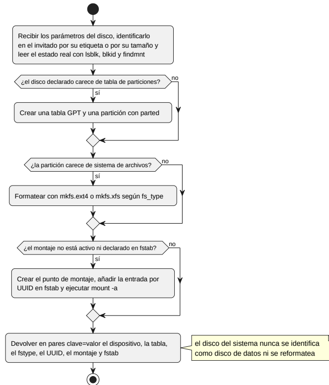
Figura 6: Diagrama de flujo de las tres guardas idempotentes de la convergencia en el invitado: cada pregunta decide si la rama sí aplica la acción o si la rama no la omite y continúa a la siguiente guarda
