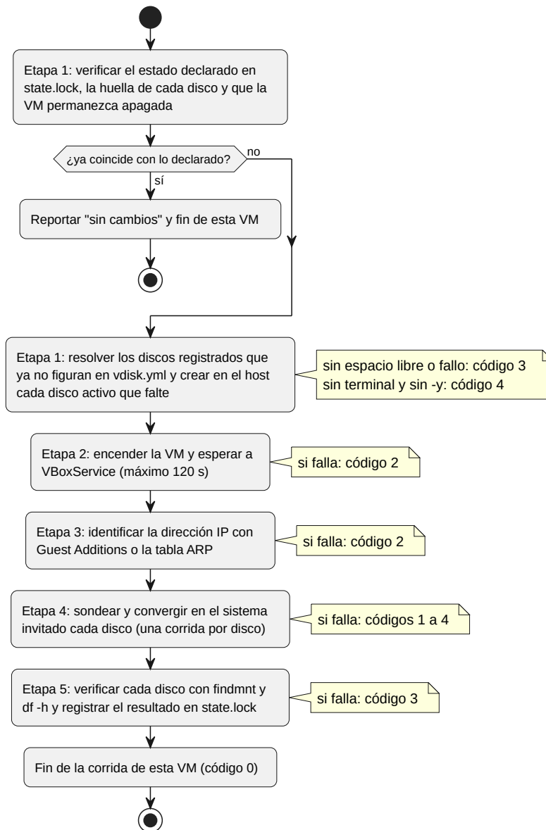
Figura 5: Diagrama de flujo de las cinco etapas de convergencia de apply por VM , con la decisión temprana de la verificación declarativa y, a la derecha de cada etapa, el código de salida cuando esta falla
