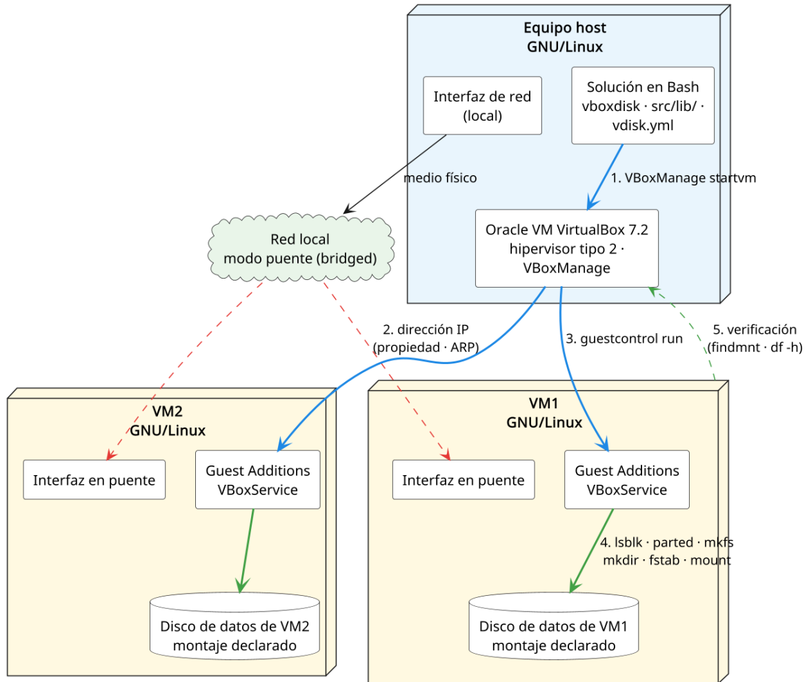
Figura 1: Escenario de despliegue: host , VirtualBox, red en modo puente, VM y almacenamiento adicional
