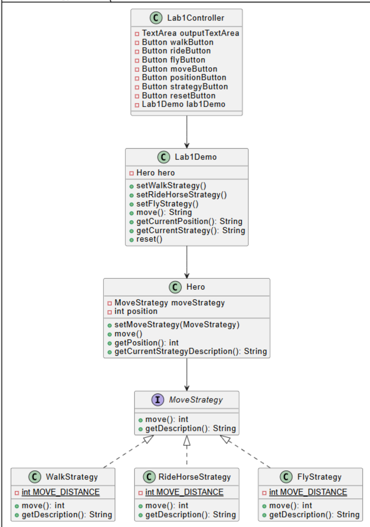
Рисунок 1 – диаграмма классов лабораторной 1
