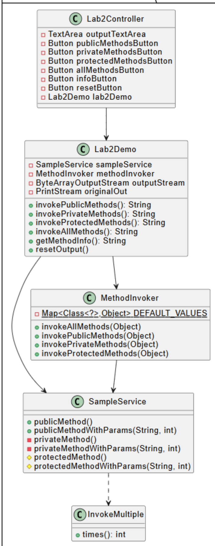
Рисунок 2 – диаграмма классов лабораторной 2
