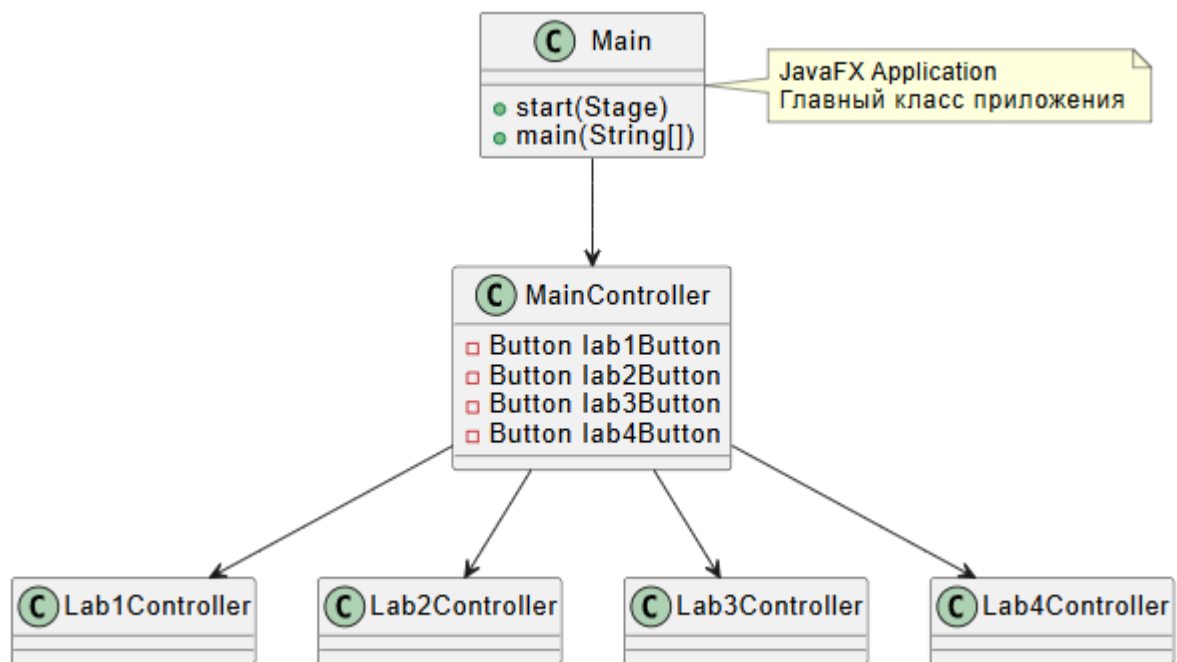
Рисунок 5 – диаграмма классов общей архитектуры приложения
