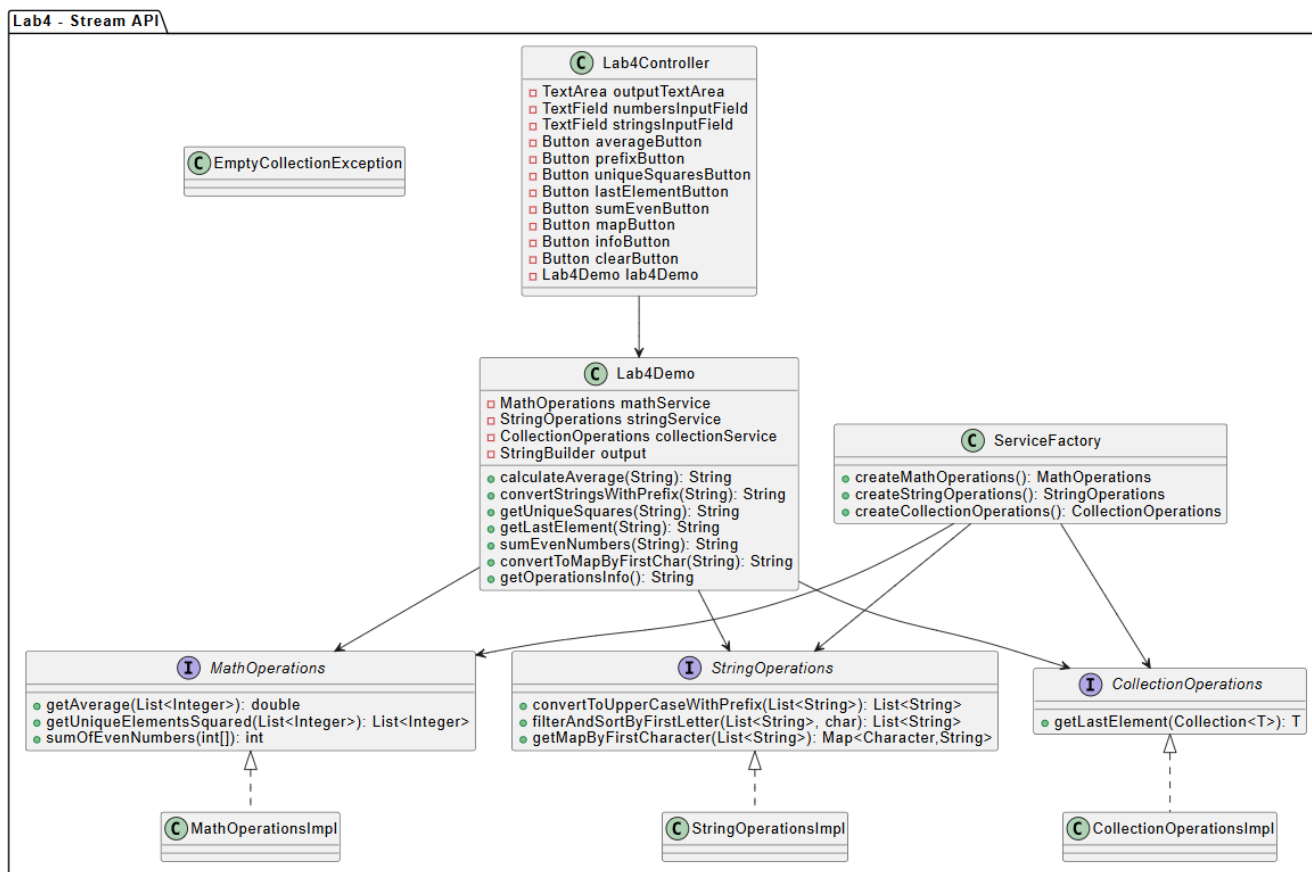
Рисунок 4 – диаграмма классов лабораторной 4
