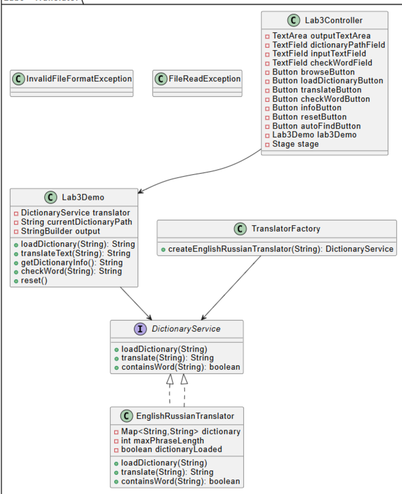
Рисунок 3 – диаграмма классов лабораторной 3
