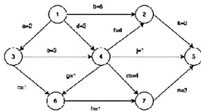
题 42 图 AOE 网络图
