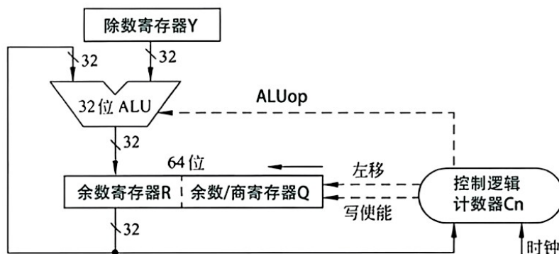
题 44 (b) 图 补码除法器逻辑结构
