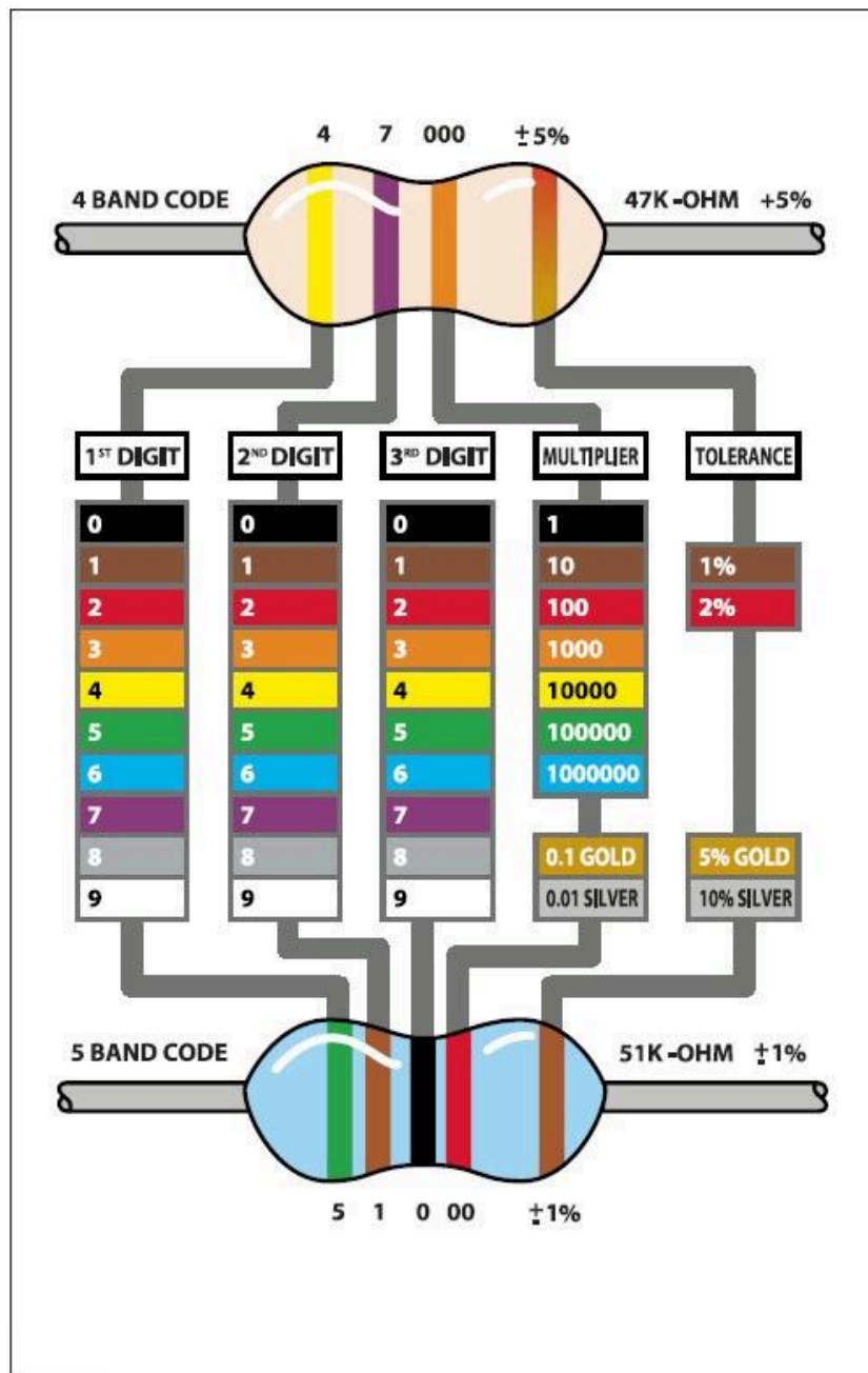
Färgkodstabell. För 4-band: digit-digit-multiplikator-tolerans. För 5-band (1 %-precision): digit-digit-digit-multiplikator-tolerans. Räkna banden innan du börjar dekodera.
