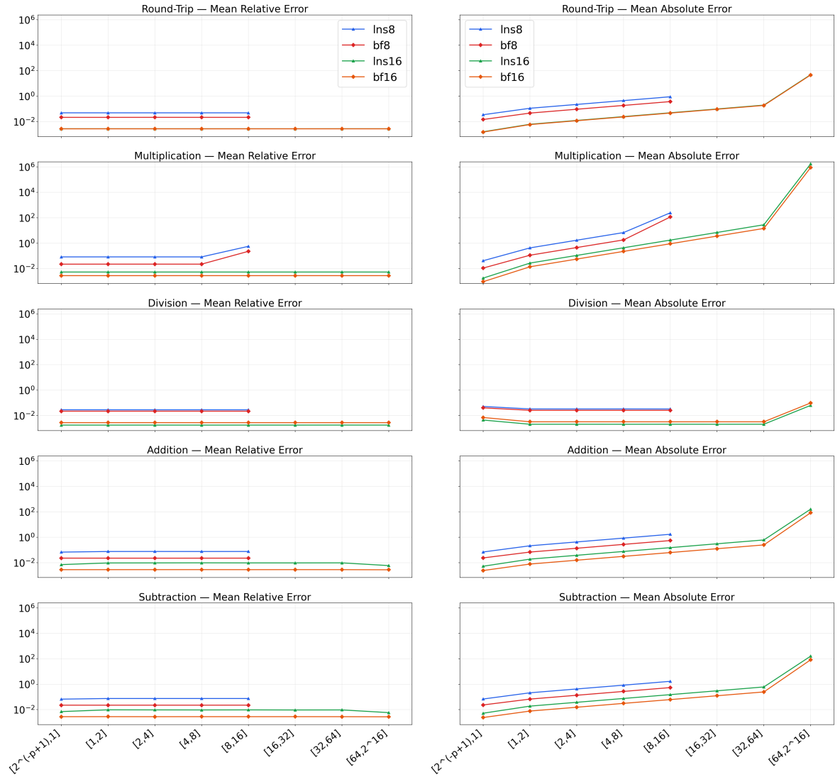
Figura 2: Erro relativo e absoluto médio por intervalo para cada operação e par de formatos. ( p é o número de bits da parte inteira do expoente em LNS — 2^{-p+1} é o número mais pequeno que ambos os formatos conseguem representar)
