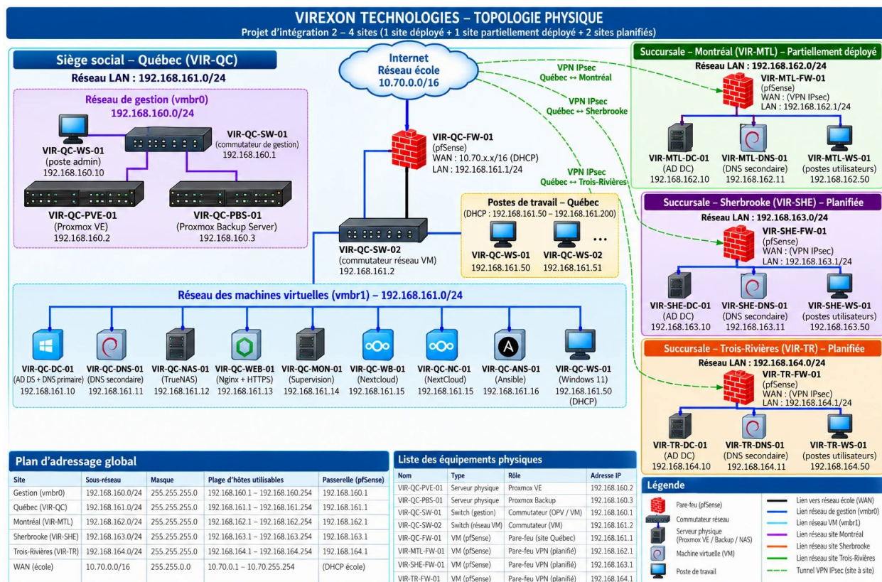
Figure 1 — Topologie physique de VIREXON Technologies
