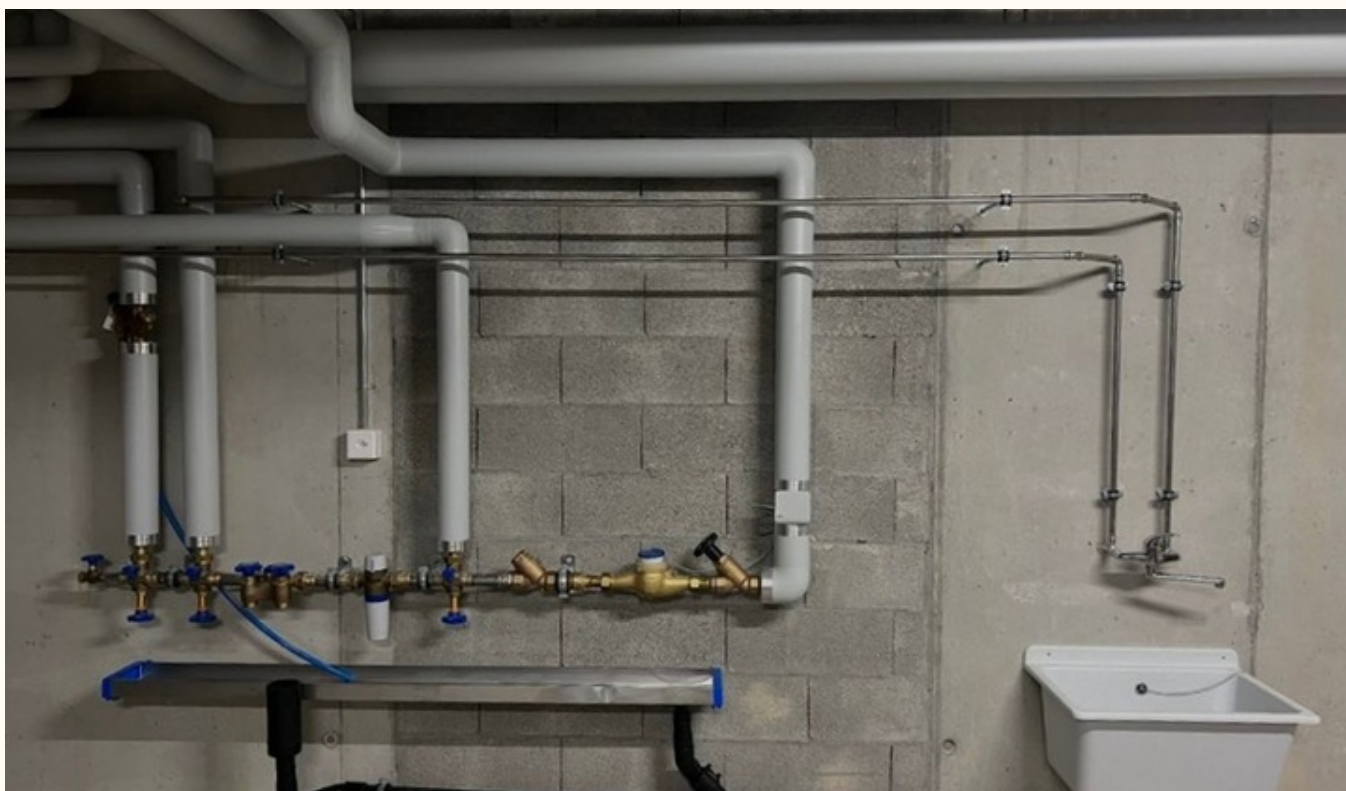
RÉSEAUX SANITAIRES
