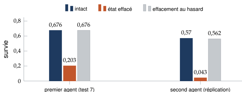
FIGURE 4 Effacer l'état fait chuter la survie ; effacer au hasard ne change rien.
