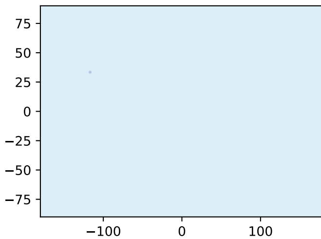
LLaVA-1.6
