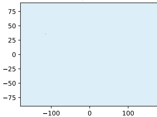
LLaVA-1.6 (SFT)
