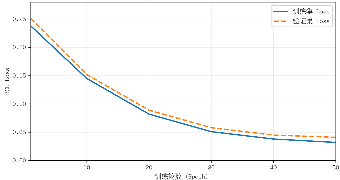
Liquid 模型训练与验证损失变化
