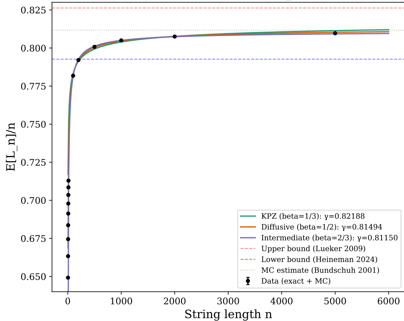
Finite-size scaling of E[L_n]/n
