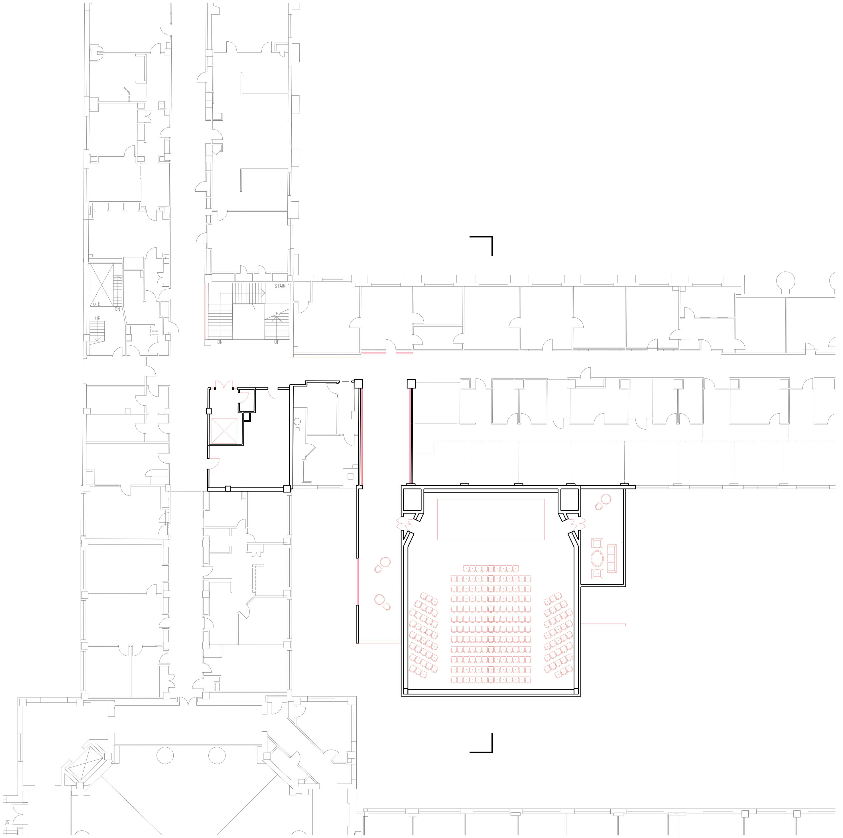
Plan 1/16"=1'
