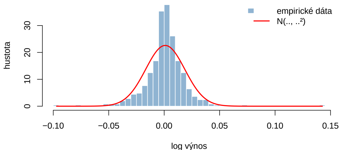
Obrázok 3: Histogram denných logaritmických výnosov AAPL s nadprispôsobenou normálnou hustotou (červená čiara). Empirické dáta vykazujú výraznejšie chvosty než predpokladá normálne rozdelenie — znak tzv. fat tails , dobre známy problém Black-Scholesovho modelu.
