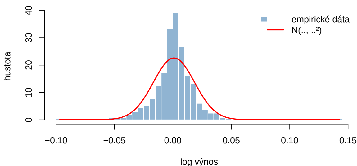
Obrázok 3: Histogram denných logaritmických výnosov AAPL s nadprispôsobenou normálnou hustotou (červená čiara). Empirické dáta vykazujú výraznejšie chvosty než predpokladá normálne rozdelenie — znak tzv. fat tails , dobre známy problém Black-Scholesovho modelu.
