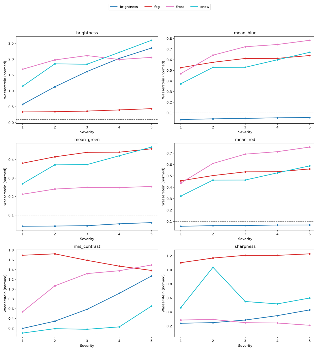
Drift (Wasserstein) vs severità — categoria: weather
