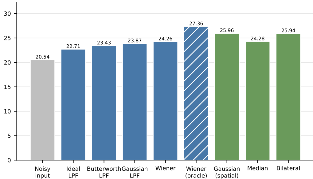
PSNR (dB)
