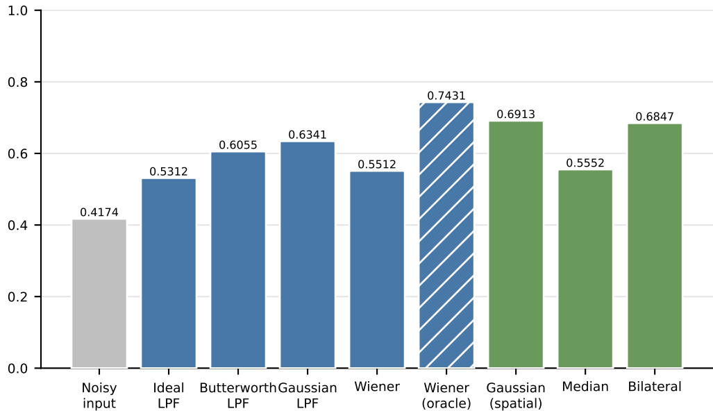
SSIM
