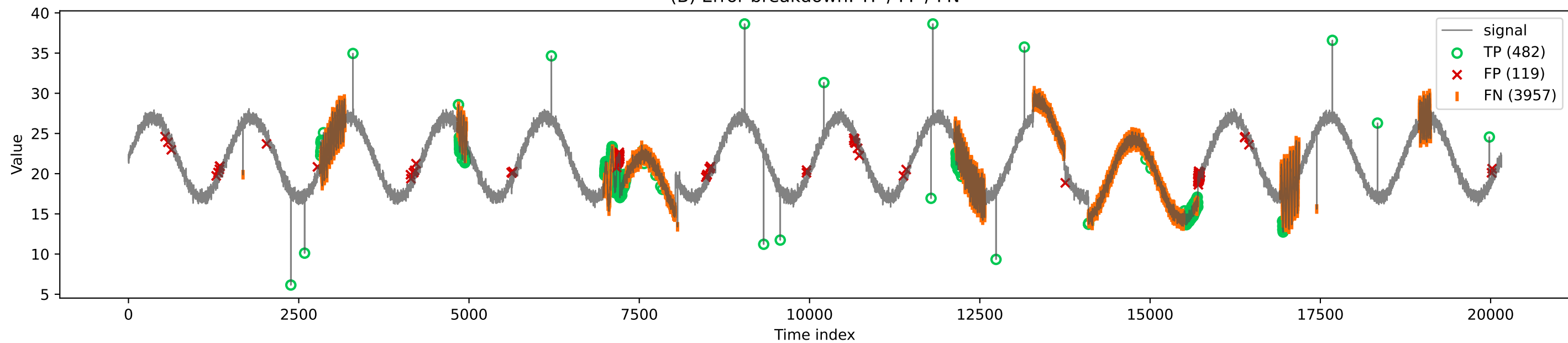
(B) Error breakdown: TP / FP / FN
