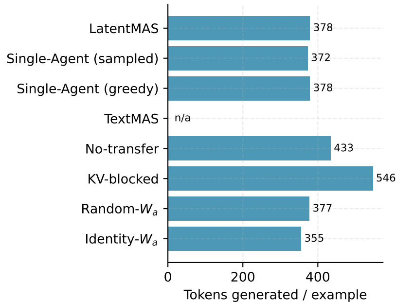
GSM8K
